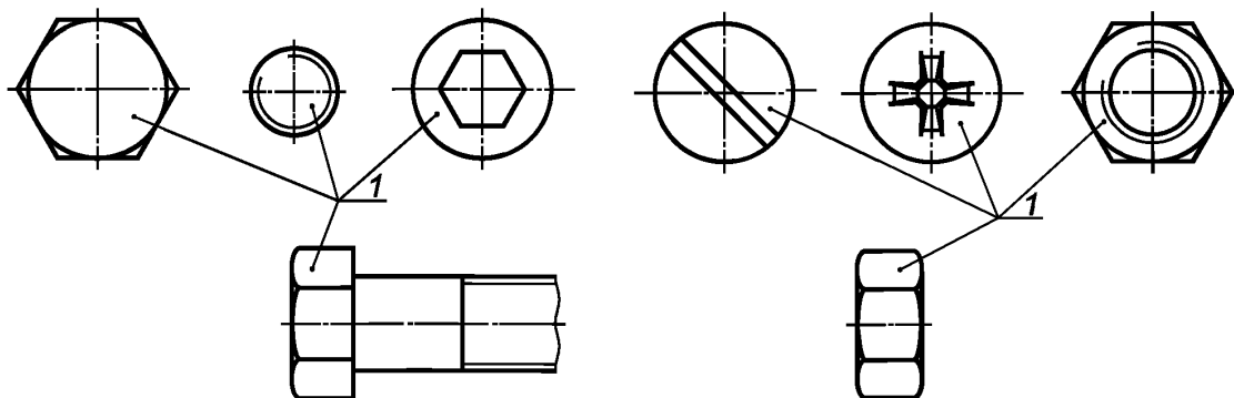
Рисунок 1 — Поверхности измерения локальной толщины покрытия на крепежных изделиях
