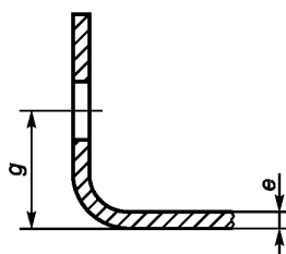
Катаный фланец
