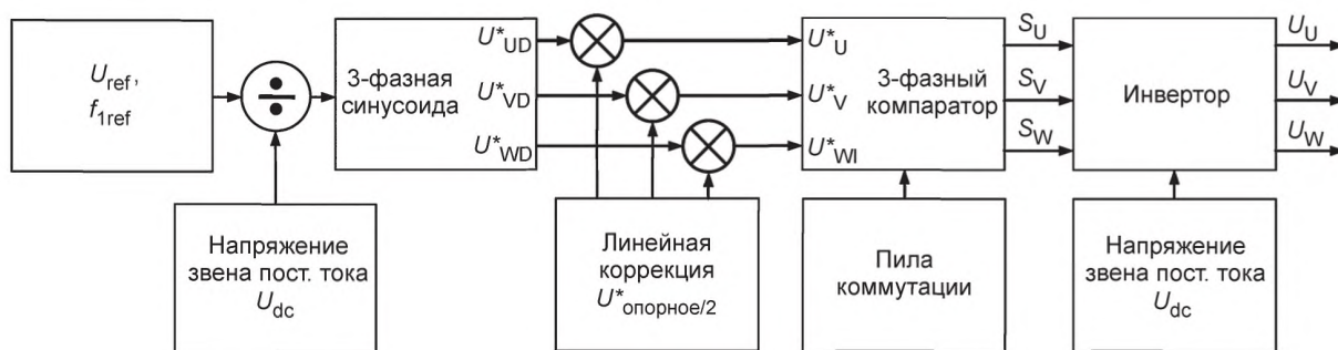
Рисунок А.2 — Структура системы формирования напряжения инвертора
