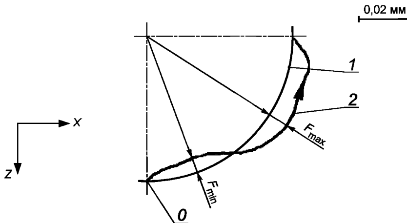
+ — центр номинальных окружностей; O — начальная точка; 1 — номинальная траектория; 2 — фактическая траектория Радиальное отклонение: F_{ZX, \max} = +0,008 мм, F_{ZX, \min} = -0,006 мм
