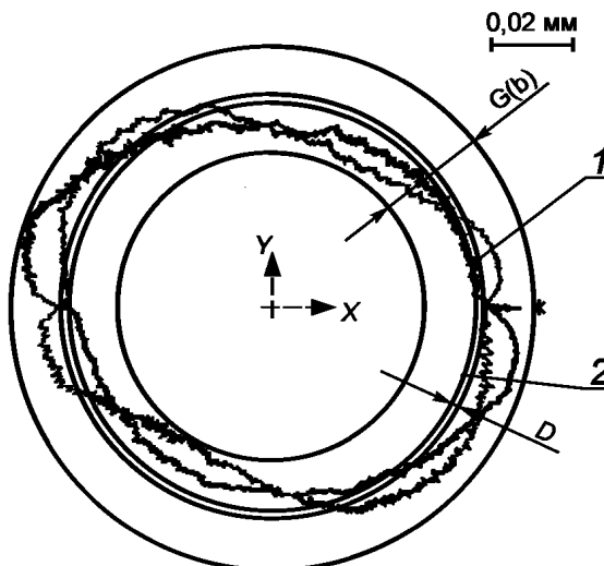
+ — центр среднеквадратичной окружности двух фактических траекторий; * — точка начала; 1 — наибольшая длина пути фактическая траектория, от +Y до +X; 2 — наименьшая длина пути фактическая траектория, от +X до +Y; двунаправленное круговое отклонение G(b)_{XY} = 0,028 мм; среднее двунаправленное радиальное отклонение D_{XY} = 0,001 мм
