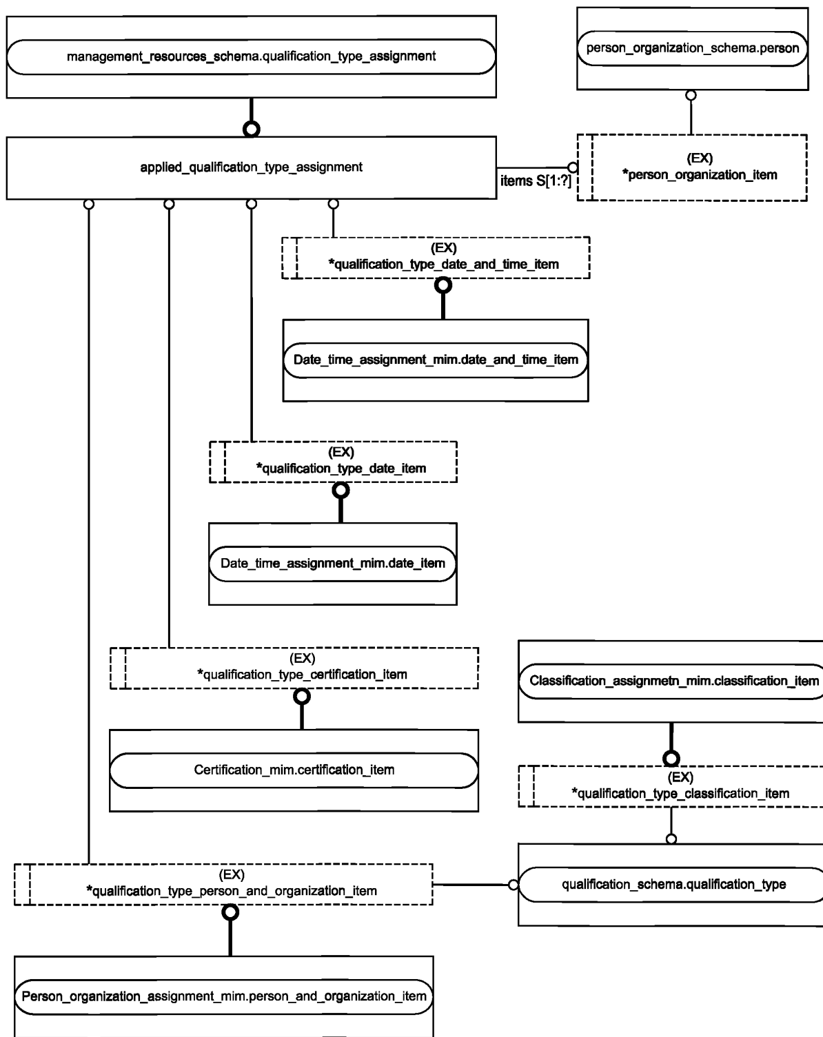
Рисунок D.2 — Представление ИММ на уровне объектов в формате EXPRESS-G
