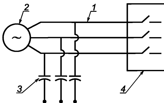
1 — питающий кабель; 2 — электродвигатель; 3 — емкость для измерений частичного разряда; 4 — размыкатель цепи
