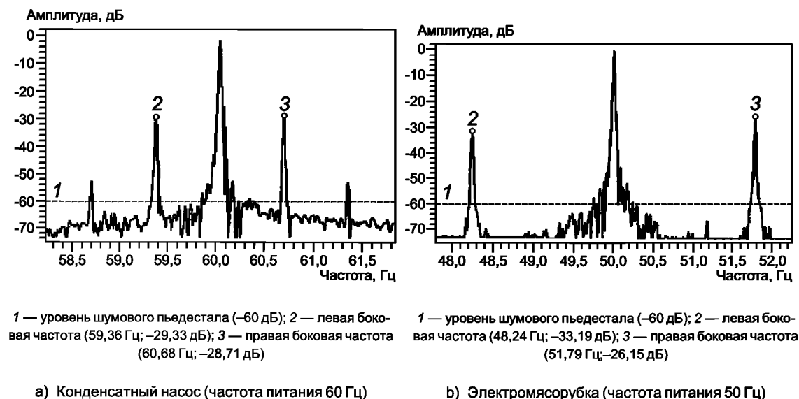
Рисунок 3 — Примеры спектров сигналов тока электродвигателей в случае обрывов стержней клетки ротора
