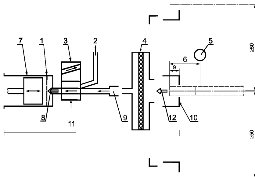
1 — положение головки поршня в начале хода; 2 — выход газовой фазы; 3 — электроклапан; 4 — ловушка для дыма; 5 — устройство для прекращения затяжки; 6 — длина окурка; 7 — насос поршневой; 8 — перемещенный объем; 9 — отверстие; 10 — держатель сигарет; 11 — канал; 12 — объем затяжки
