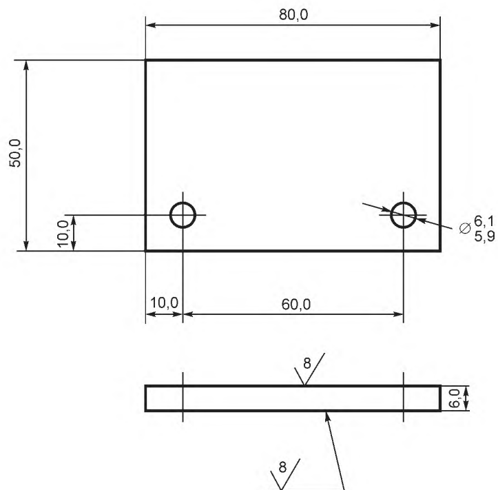
Рисунок 5 — Прижимная пластина и опорный фитинг
