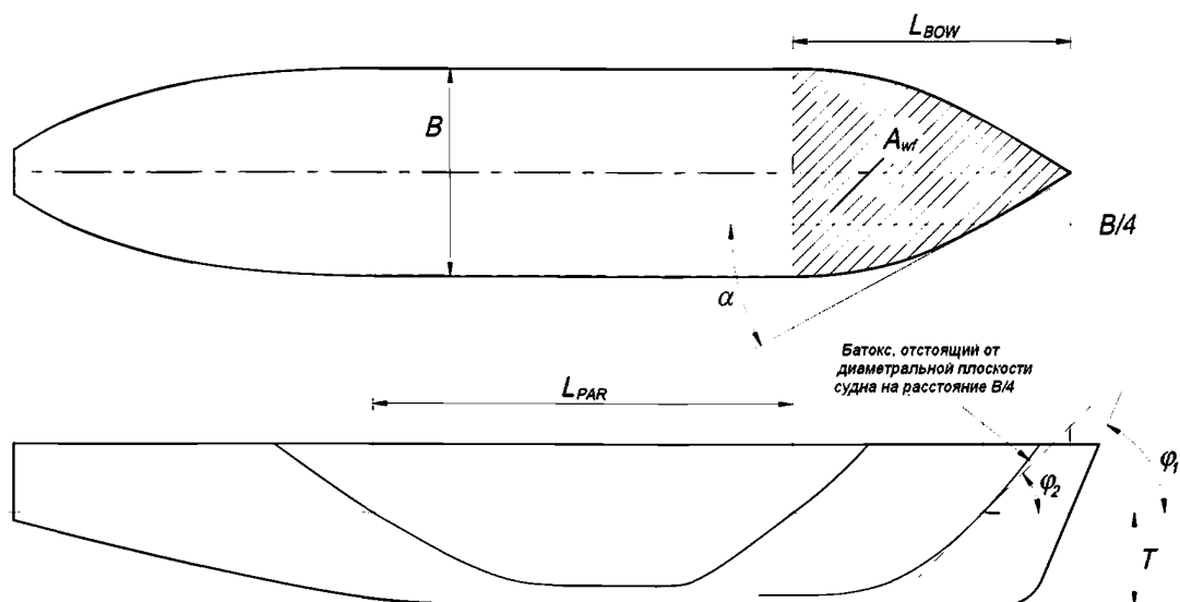
Рис. 2.1.1.4 Геометрические характеристики судна при определении мощности на гребных валах судов ледовых классов
