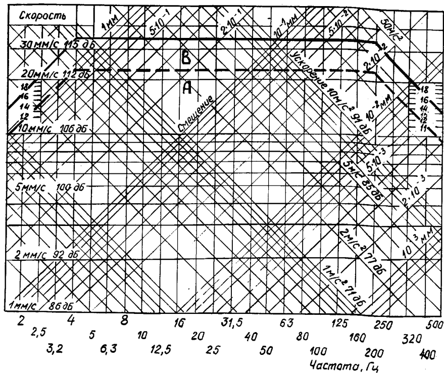
Рис. 9.3.4 Нормы вибрации турбокомпрессоров ДВС:
