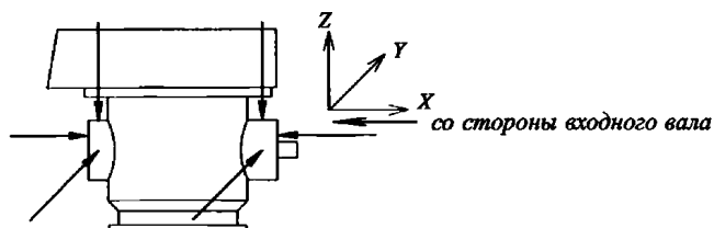
Рис. 9.9.2 Точки измерения вибрации винторулевых колонок
