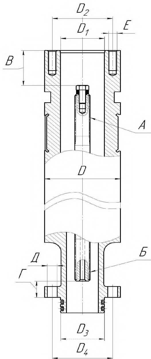
Рисунок К.1 — Габаритные и присоединительные размеры гидрозащит с диаметром корпуса 69; 81; 86; 92; 103; 114 мм
