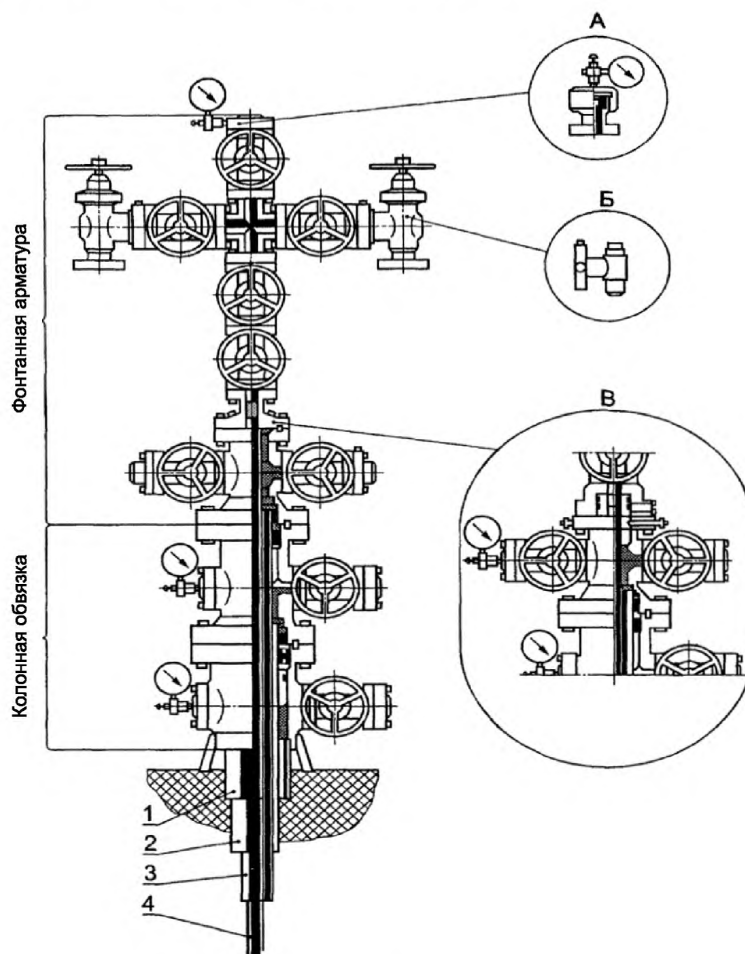
А — буферный фланец под устьевой герметизатор; Б — регулируемый дроссель; В — подвеска НКТ и скважинной насосной установки в трубной головке (на муфте); 1 — кондуктор; 2 — техническая колонна; 3 — эксплуатационная колонна; 4 — колонна НКТ и скважинное оборудование
