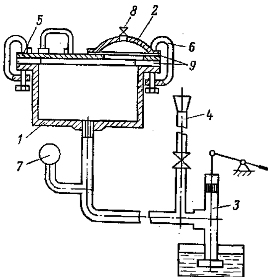
Рис. 6. Принципиальная схема устройства для гидравлических испытаний деталей оболочек, имеющих отверстия для выхода воздуха при заполнении их водой:
