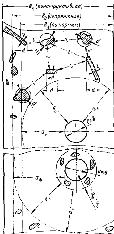
Рис. 1. Разделки пороков литья и следов механических повреждений:
