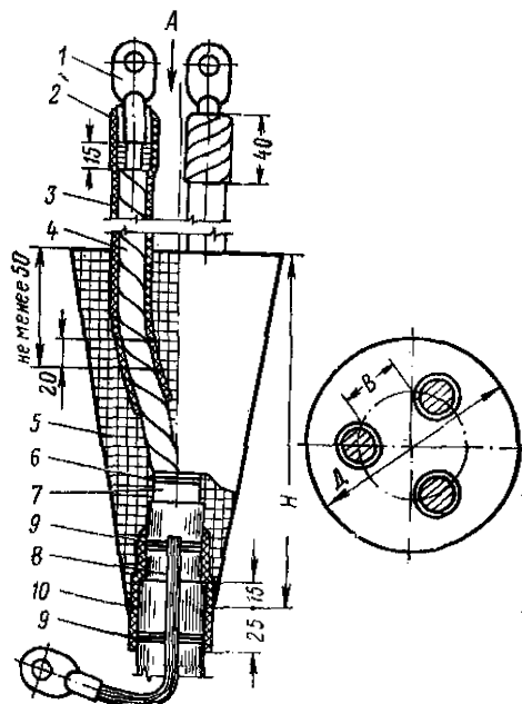
Рис 4. Общий вид эпоксидной заделки с трехслойными трубками:
