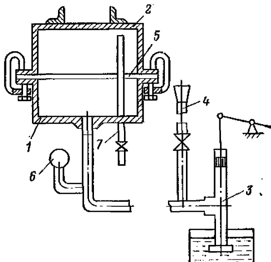
Рис. 5. Принципиальная схема устройства для гидравлических испытаний деталей оболочек, не имеющих отверстия для выхода воздуха при заполнении их водой:
