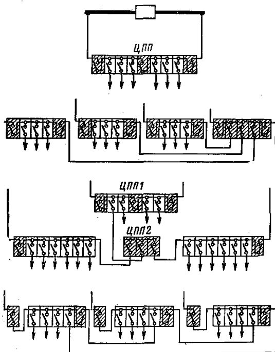
Рис. 1. Примерные схемы расстановки аппаратов в ЦПП
