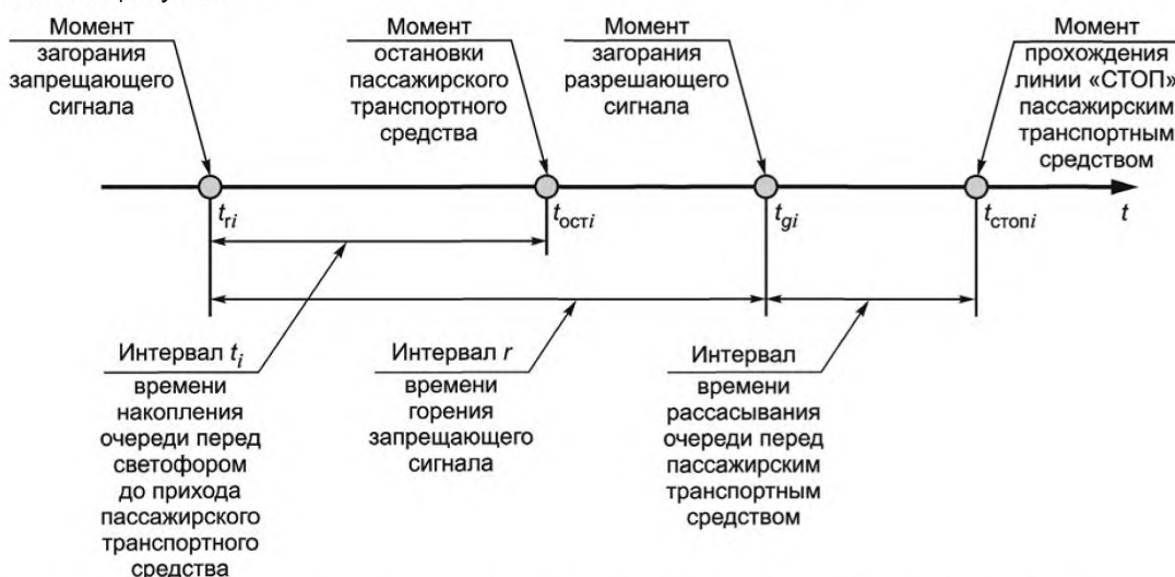
Рисунок 5 — Последовательность основных событий, рассматриваемых при расчетах интенсивности движения транспортных средств на полосе движения пассажирского транспортного средства
