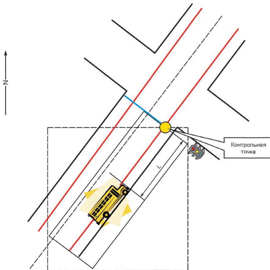
Рисунок 4 — Схема организации пространственной модели регулируемого перекрестка
