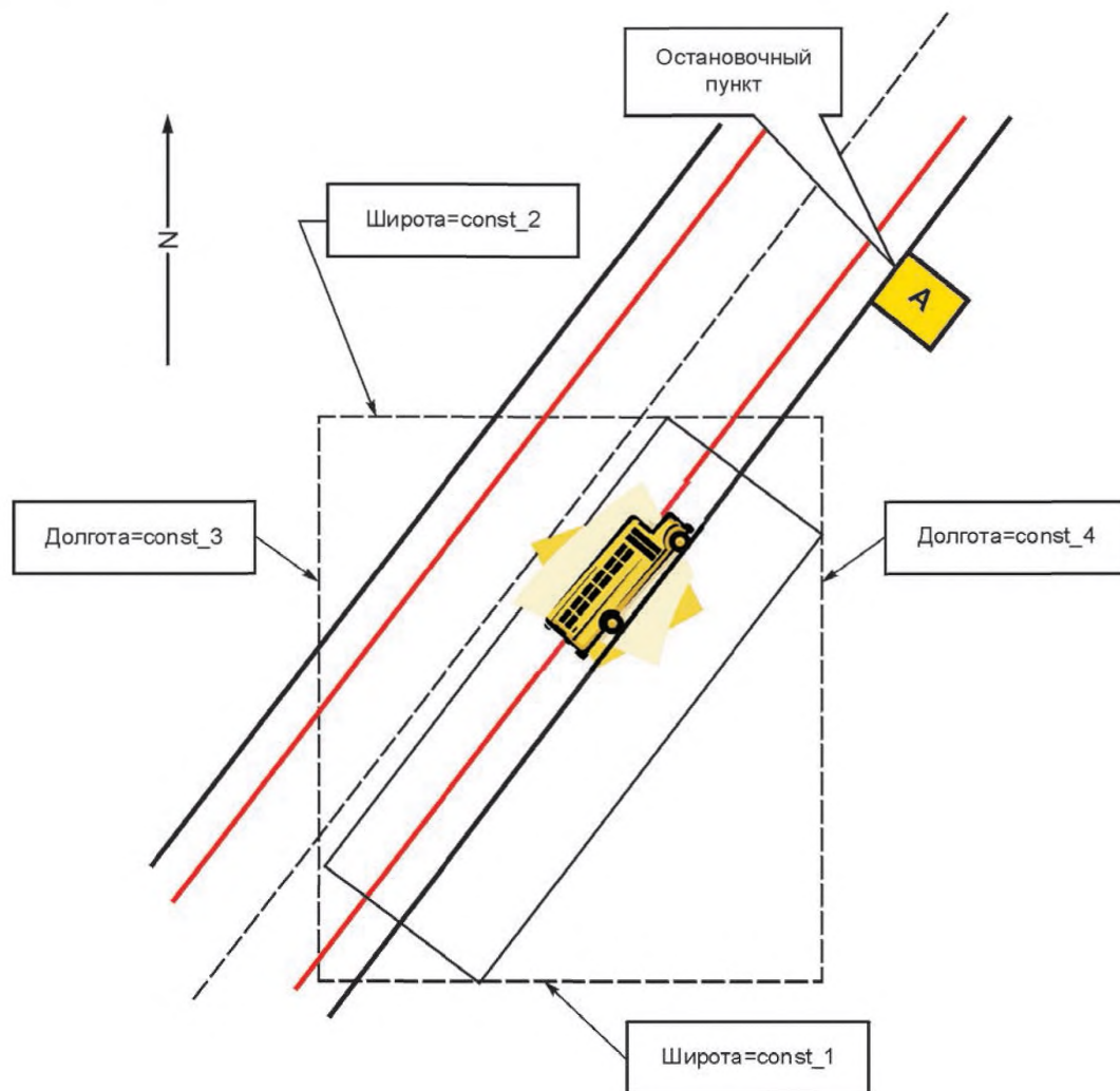
Рисунок 2 — Схема организации пространственной модели участка
