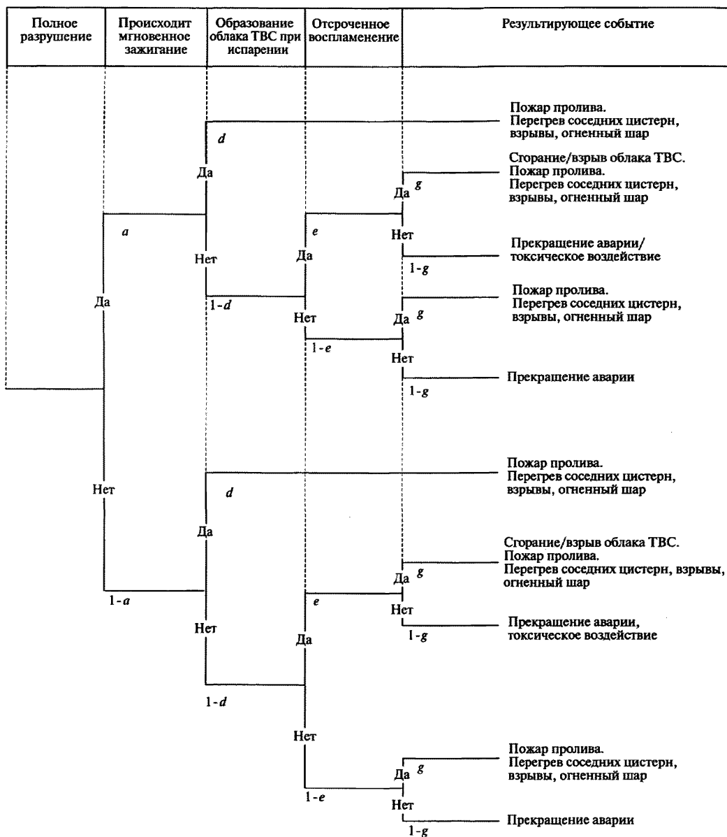
Рис. 4-2. Дерево событий при сходе (разрушении) цистерны (группы цистерн), содержащей (содержащих) продукт при атмосферном давлении
