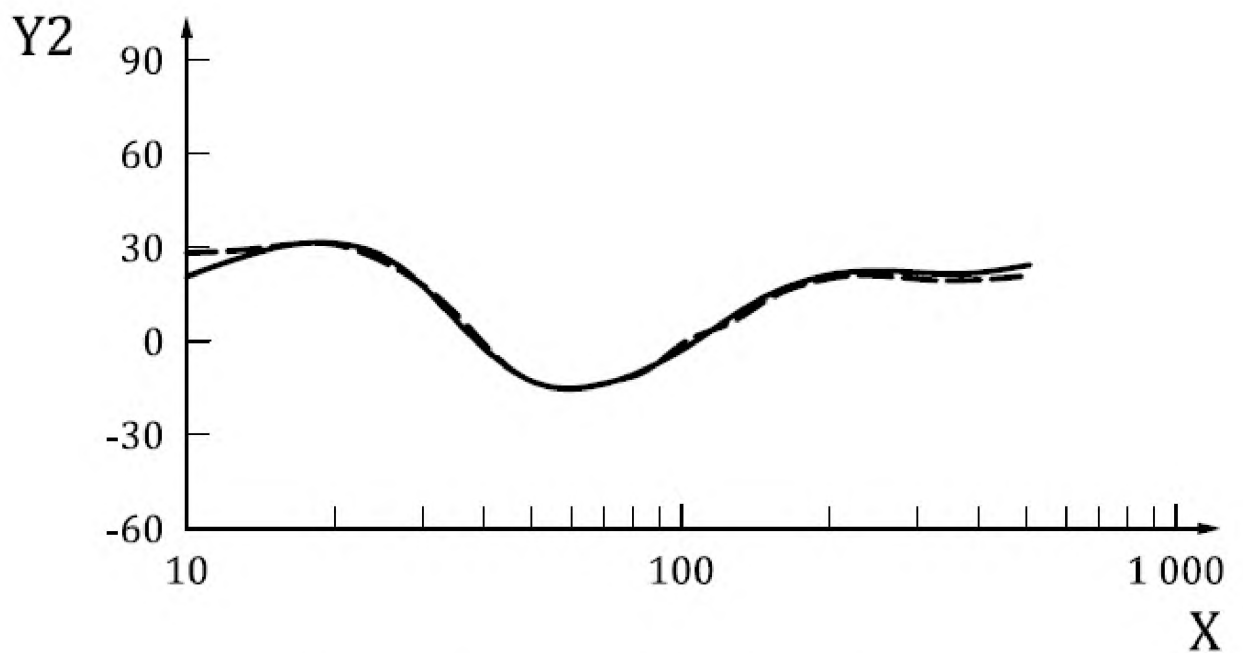
Рисунок С.4 — Сравнение результатов моделирования (сплошная линия) и опорных значений (пунктирная линия) механического импеданса системы «кисть — рука» в направлении Z_{11}
