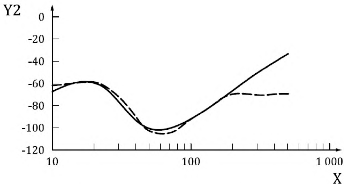
Рисунок В.4 — Сравнение результатов моделирования (сплошная линия) и опорных значений (пунктирная линия) эффективной массы системы «кисть — рука» в направлении z_1
