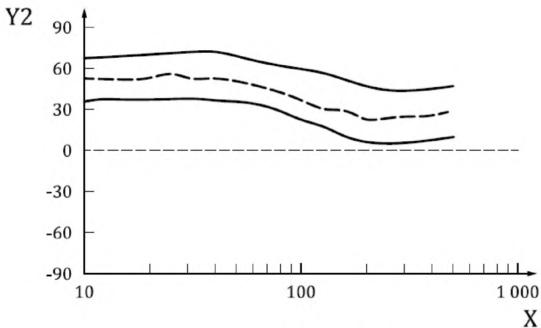
Рисунок 1 — Значения входного механического импеданса для системы «кисть — рука» в направлении x_1
