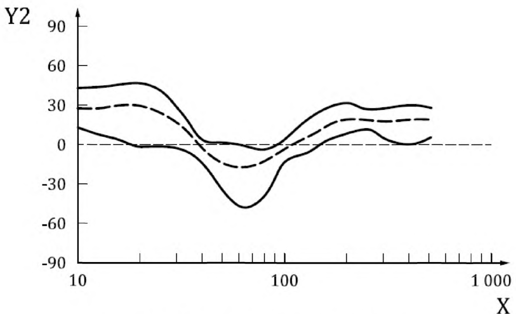
Рисунок 3 — Значения входного механического импеданса для системы «кисть — рука» в направлении z_h
