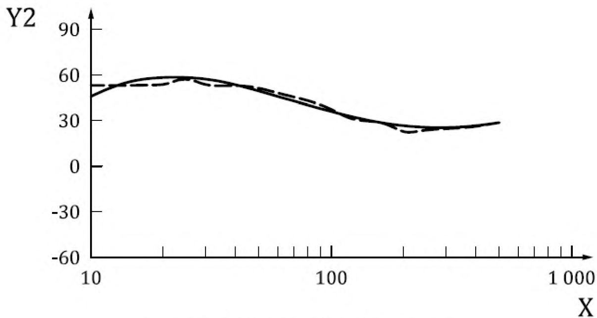
Рисунок D.2 — Сравнение результатов моделирования (сплошная линия) и опорных значений (пунктирная линия) механического импеданса системы «кисть — рука» в направлении x_h
