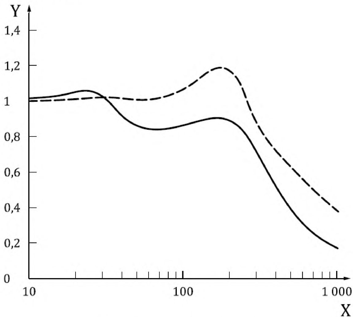
Рисунок Е.2 — Предсказанный моделью коэффициент передачи перчаток в области пальцев (сплошная линия) и ладони (пунктирная линия) в направлении z_h
