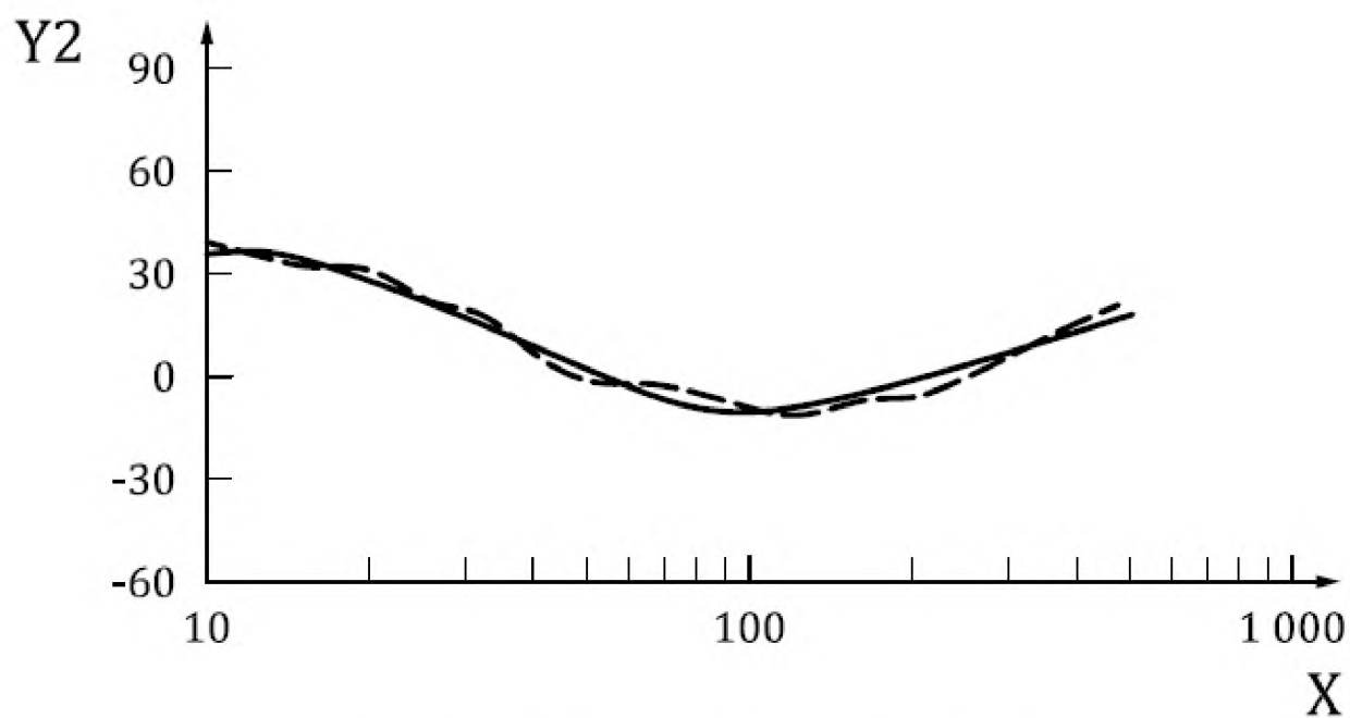
Рисунок D.3 — Сравнение результатов моделирования (сплошная линия) и опорных значений (пунктирная линия) механического импеданса системы «кисть — рука» в направлении y_h
