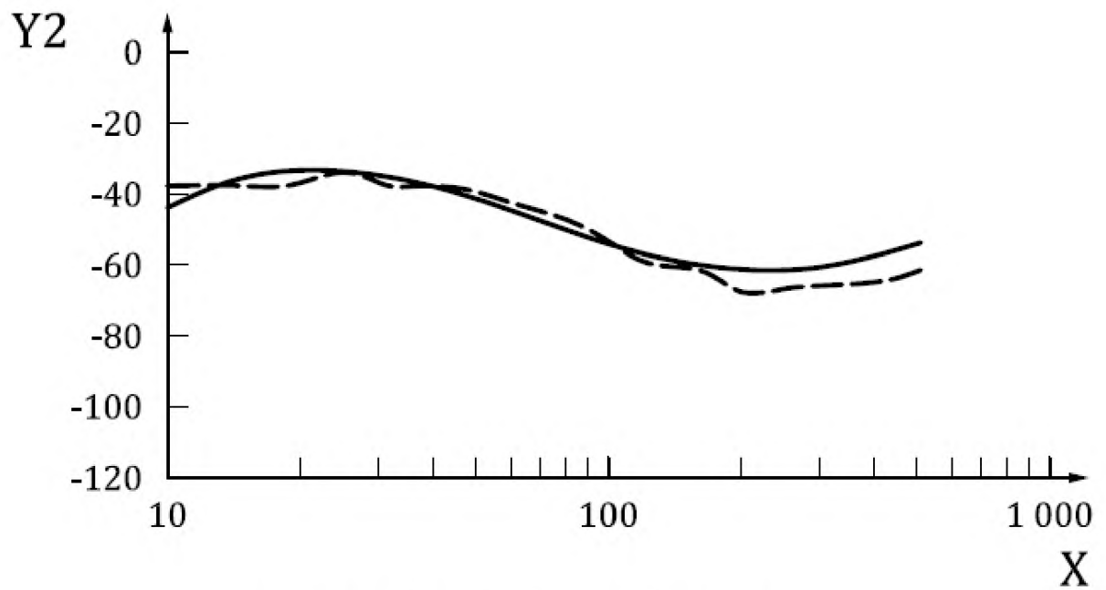
Рисунок В.2 — Сравнение результатов моделирования (сплошная линия) и опорных значений (пунктирная линия) эффективной массы системы «кисть — рука» в направлении x_h
