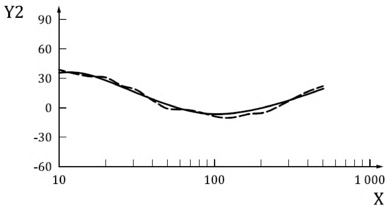
Рисунок С.3 — Сравнение результатов моделирования (сплошная линия) и опорных значений (пунктирная линия) механического импеданса системы «кисть — рука» в направлении y_h
