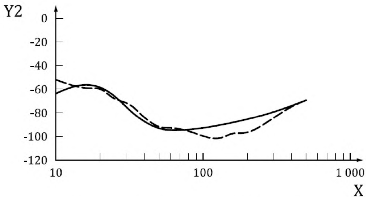
Рисунок В.3 — Сравнение результатов моделирования (сплошная линия) и опорных значений (пунктирная линия) эффективной массы системы «кость — рука» в направлении Y_h
