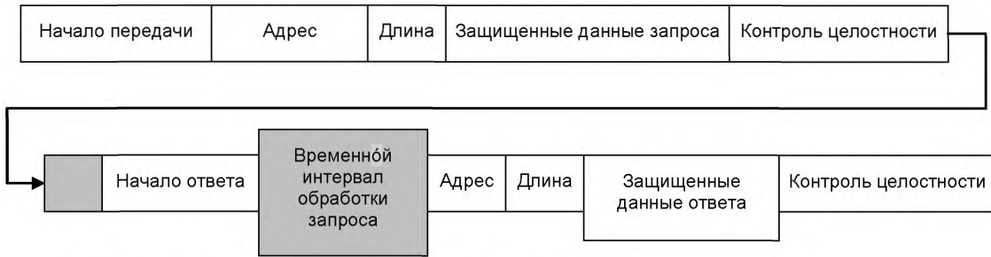
Рисунок 1 — Пример структуры обмена сообщениями в объектовом интерфейсе
