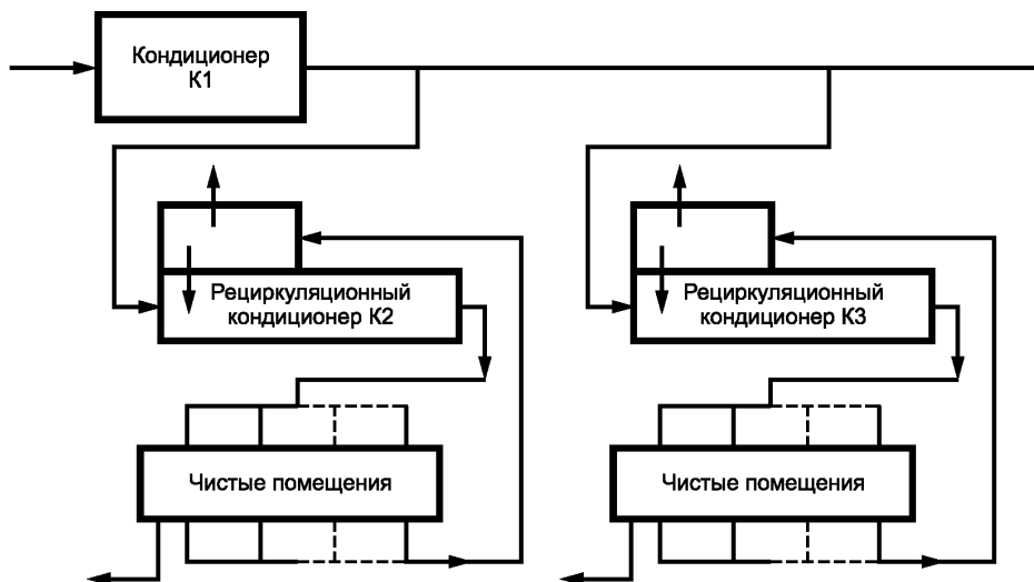
Рисунок А.4 — Двухуровневая система вентиляции и кондиционирования
