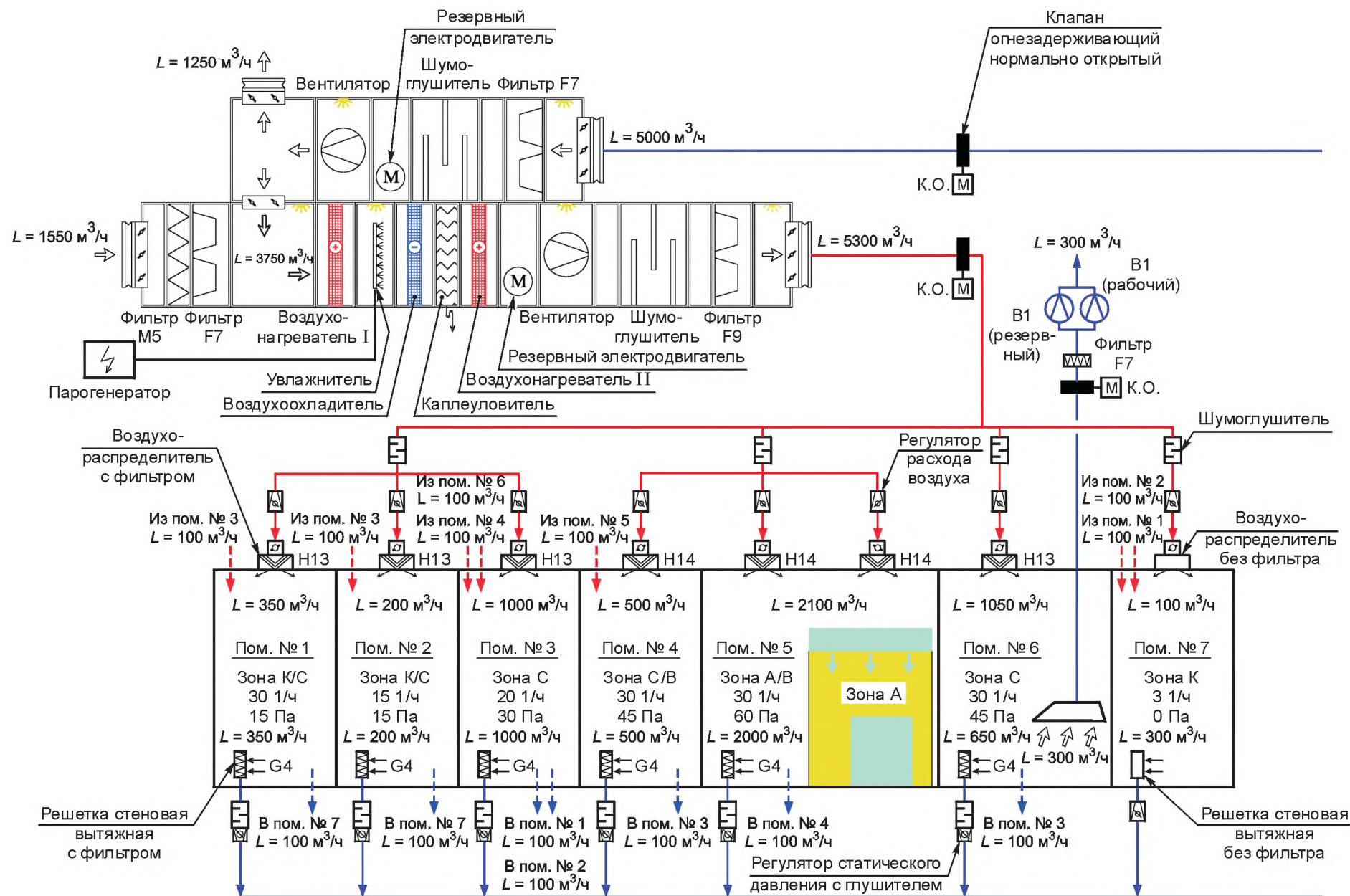
Рисунок В.1 – Пример принципиальной схемы вентиляции и кондиционирования воздуха
