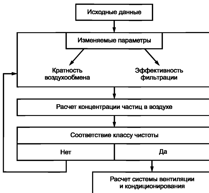
Рисунок С.2 — Подбор кратности воздухообмена в зависимости от класса чистоты и эффективности фильтрации воздуха
