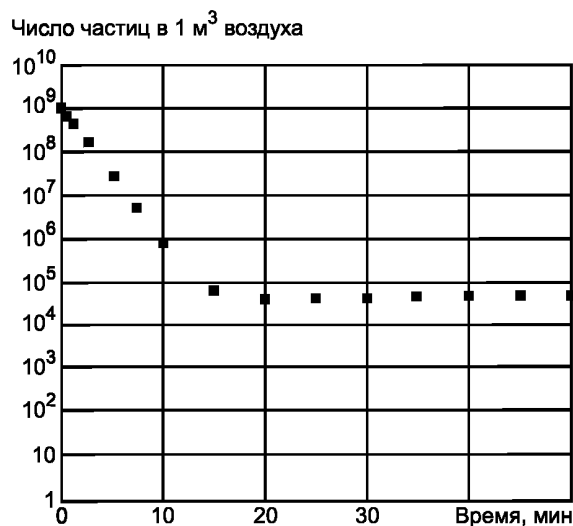
Рисунок С.1 — Зависимость концентрации частиц от времени после пуска чистого помещения
