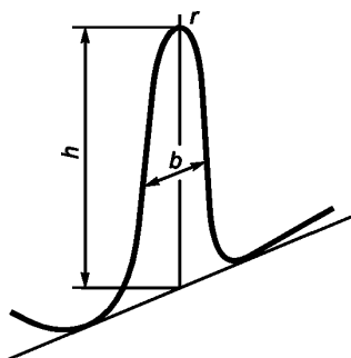
Рисунок 1 — Пик на хроматограмме
