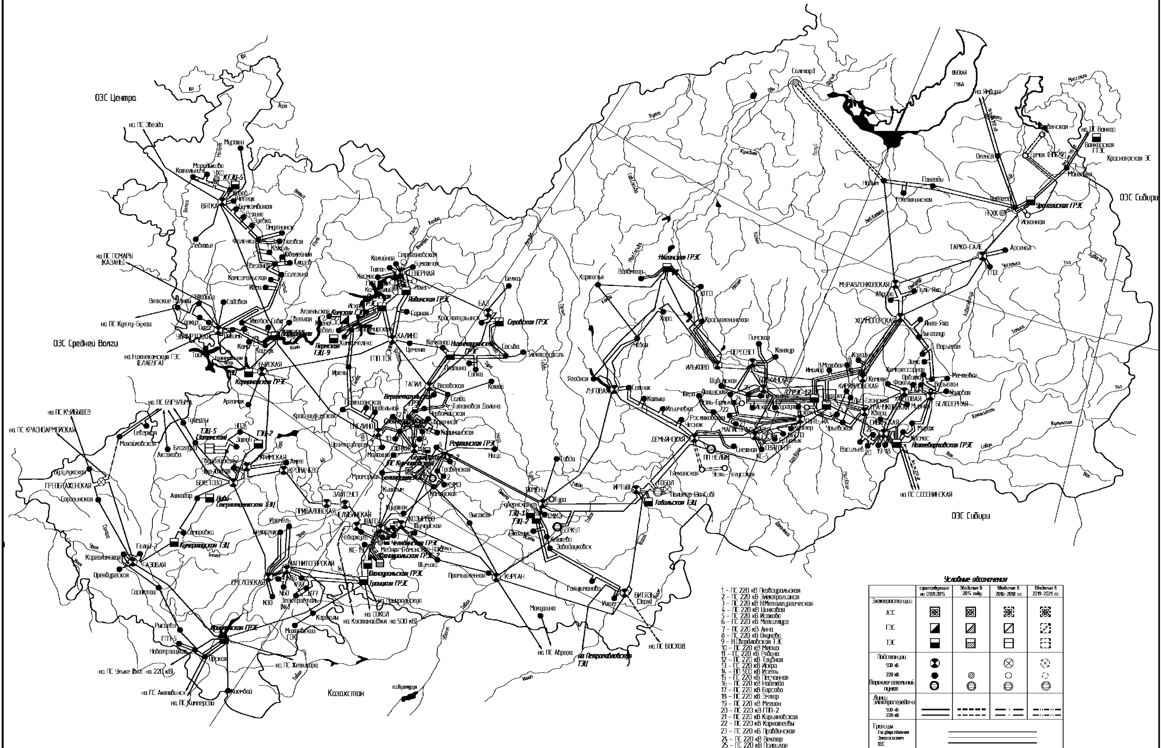
Карта-схема размещения линий электропередачи, подстанций напряжением 220 кВ и выше и электростанций ОЭС Урала на 2015-2021 годы
