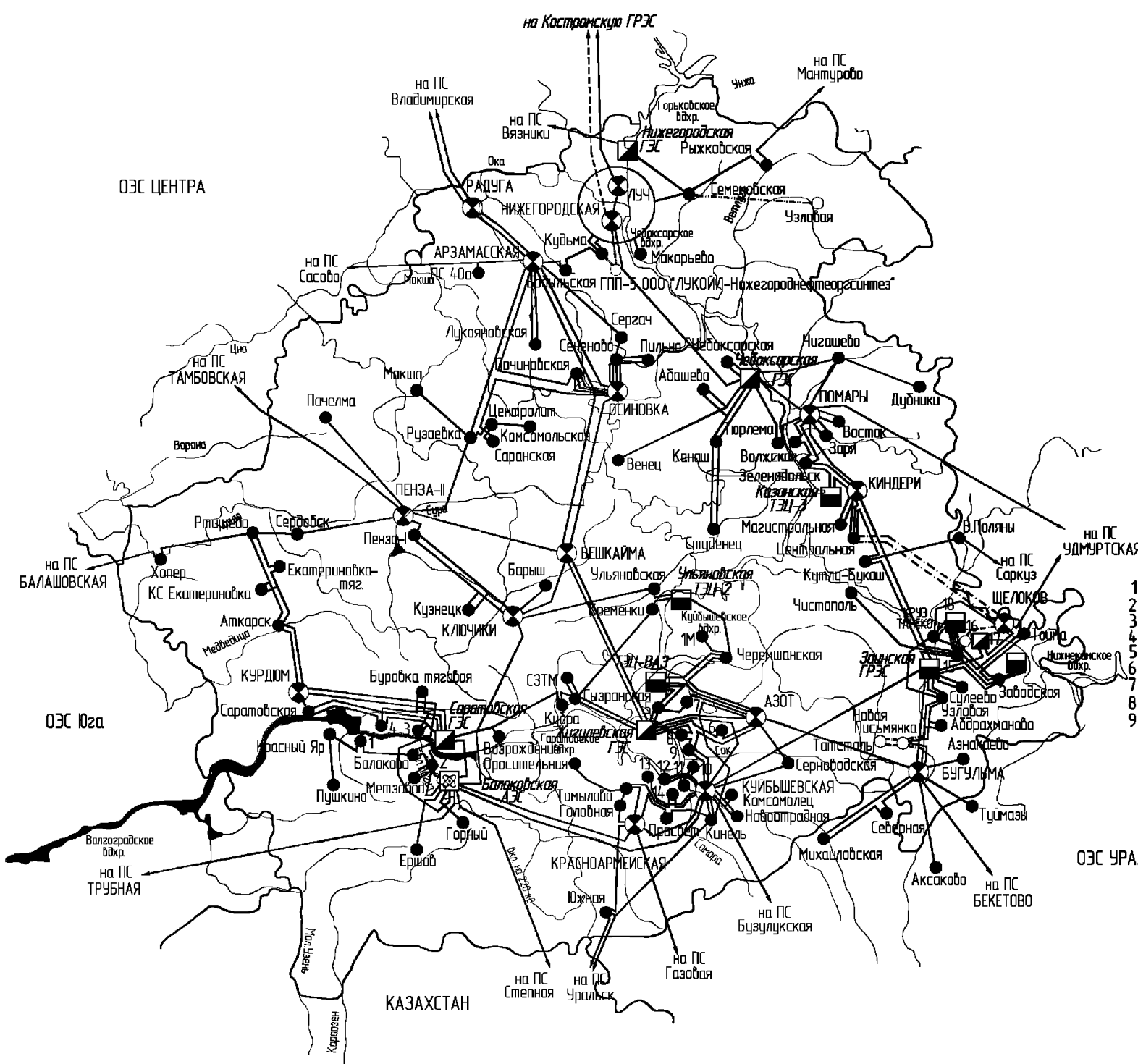
Карта-схема размещения линий электропередачи, подстанций напряжением 220 кВ и выше и электростанций ОЭС Средней Волги на 2015-2021 годы
