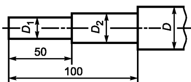
Рисунок А.1 — Форма образца
