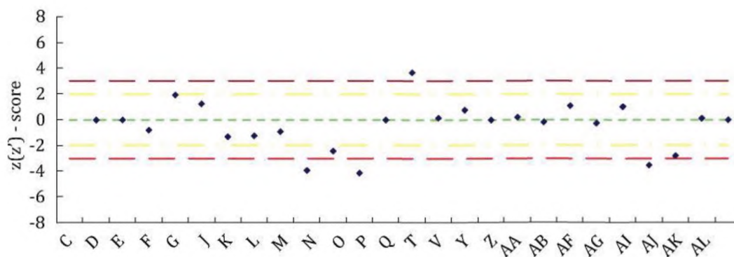
Рисунок А.3 – График Z-оценок измерения процентного содержания сухой массы вискозы
