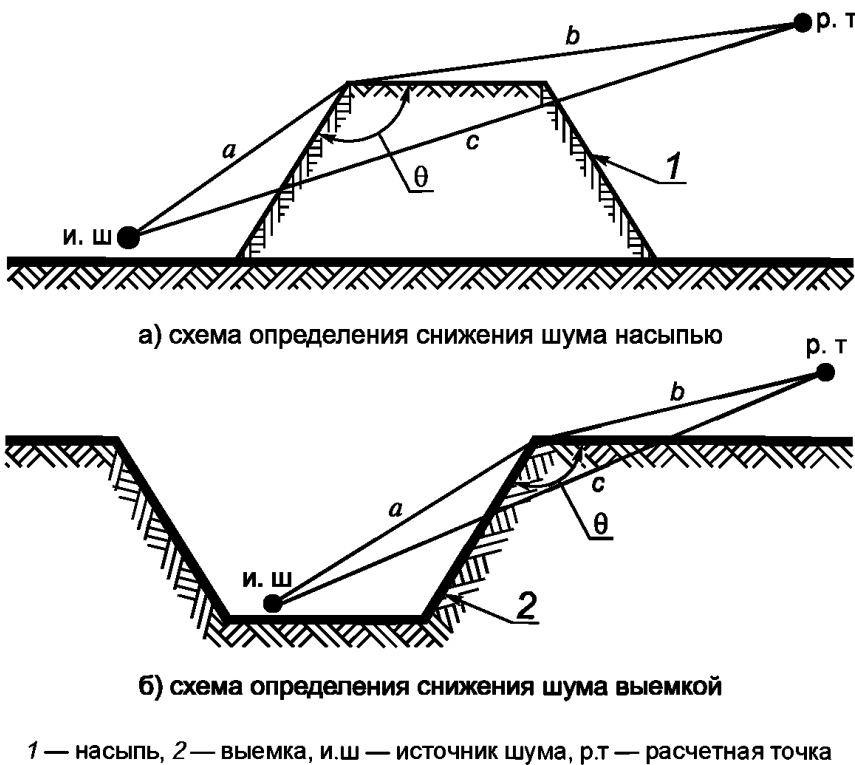
Рисунок 5 — Схема определения снижения шума
