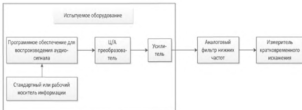
Рисунок 8 — Блок-схема измерения кратковременного искажения.
