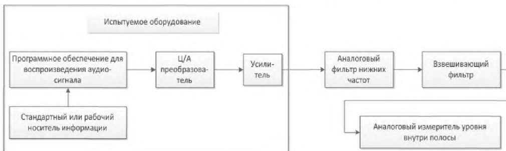
Рисунок 4 — Блок-схема для измерения отношения сигнал-шум
