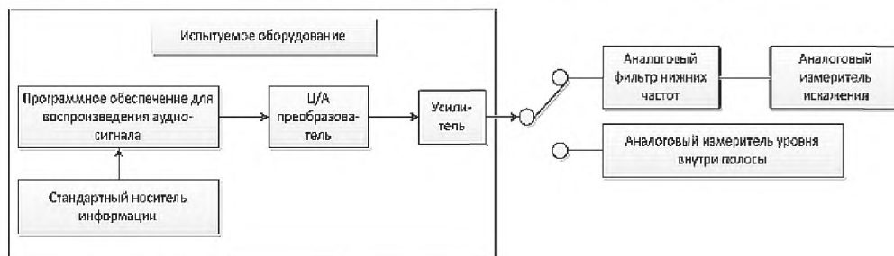
Рисунок 1 — Блок-схема для измерения максимальной амплитуды выходного сигнала
