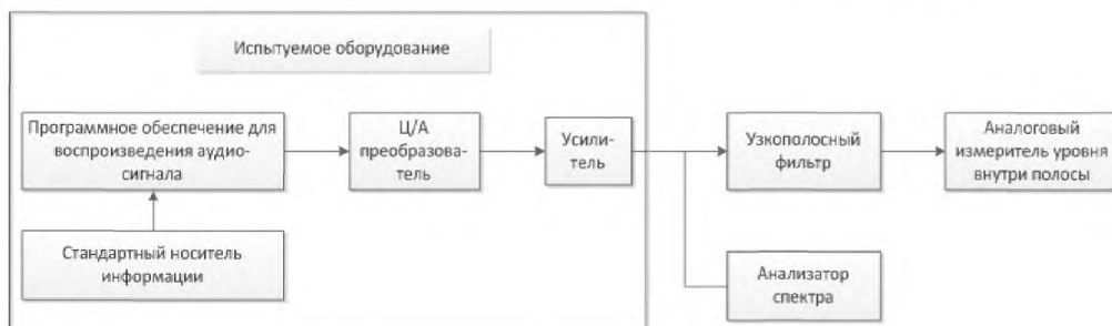
Рисунок 6 — Блок-схема для измерения разделения каналов
