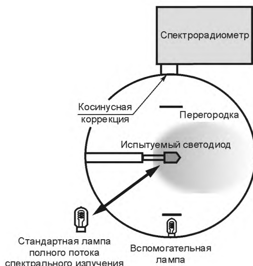
Рисунок 4 — Оптическая схема измерений в режиме полного потока
