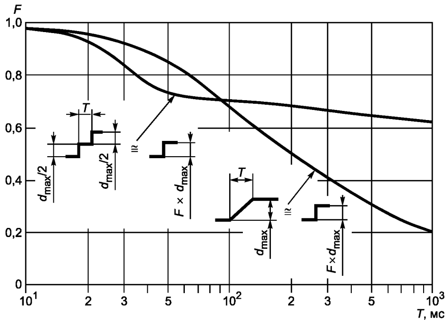
Рисунок 3 — Коэффициент формы F для двухступенчатых и линейно изменяющихся характеристик напряжения
