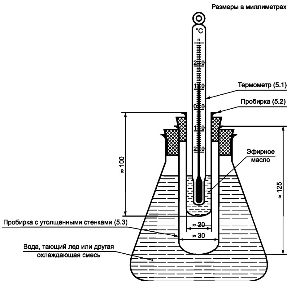
Рисунок — Подходящий прибор для определения температуры застывания
