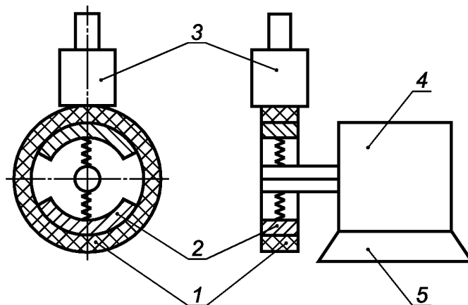
1 — контролируемое изделие; 2 — фиксирующие кулачки; 3 — ударный преобразователь; 4 — механизм позиционирования; 5 — массивное основание
