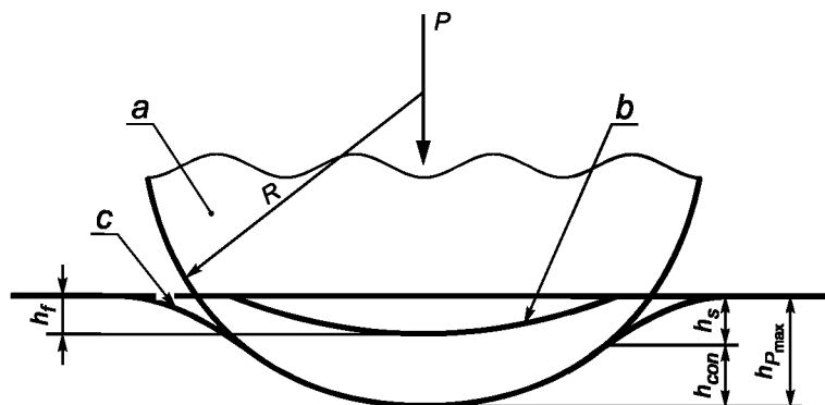
Рисунок 2 — Схематическое представление поперечного сечения лунки при деформировании материала шаровым индентором
