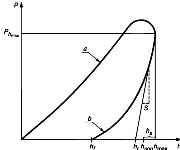
Рисунок 1 — Типичная диаграмма ударного вдавливания индентора в испытуемый материал
