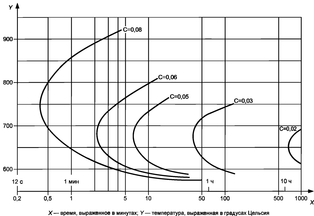
Рисунок D.1 — Температурно-временная диаграмма межкристаллитной коррозии в аустенитной нержавеющей стали марки А2
