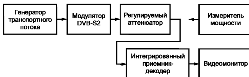
Рисунок 2 — Схема измерения чувствительности и максимального уровня принимаемого сигнала
