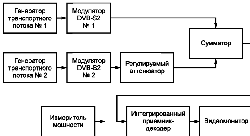
Рисунок 4 — Схема измерения избирательности по соседнему и зеркальному каналам
