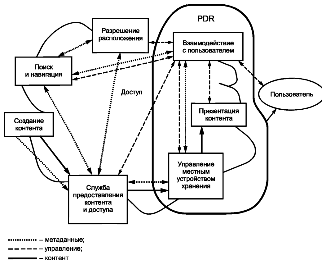
Рисунок 2 — Полная интерактивная модель системы TV-Anytime
