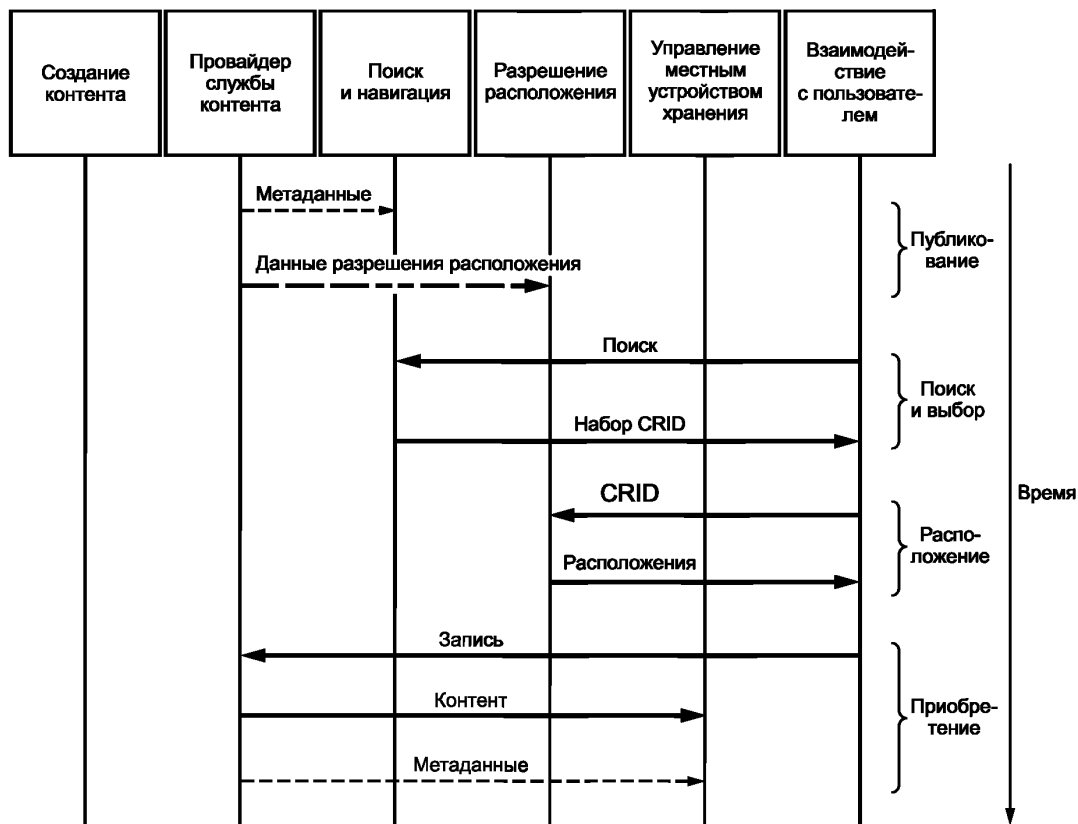
Рисунок 10 — Пример динамического поведения процессов в системе TV-Anytime
