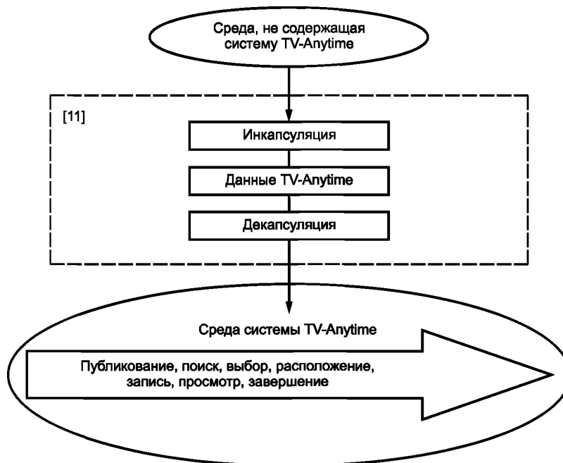
Рисунок 3 – Формат обмена данными
