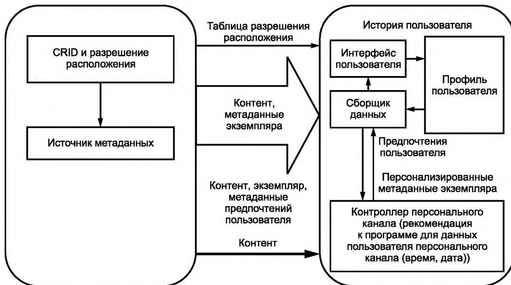
Рисунок 12 – Операции взаимодействия между провайдером служб и пользователем
