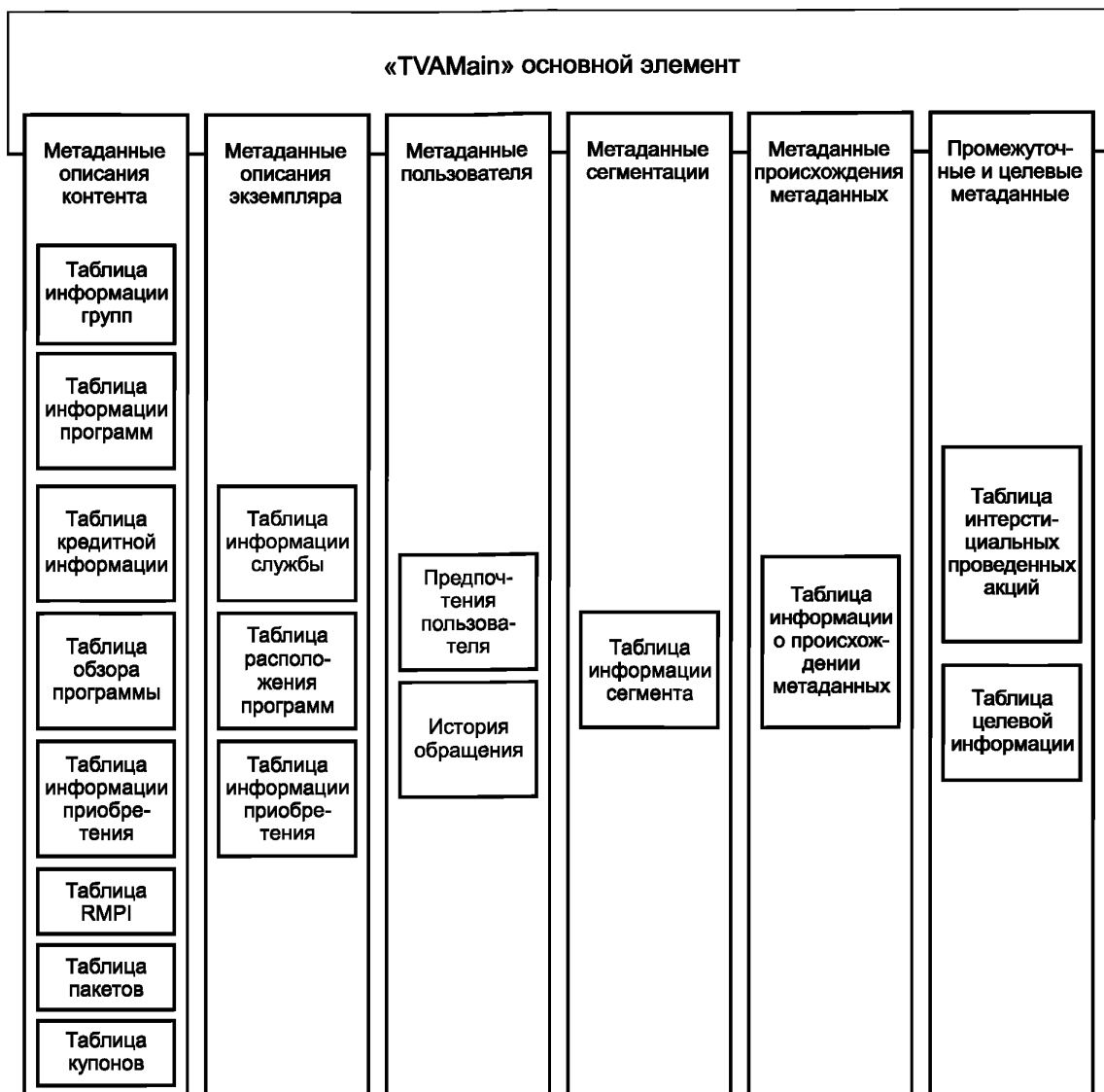
Рисунок 6 – Документы TV-Anytime с корневым элементом «TVAMain»
