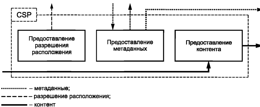
Рисунок 5 – Расширенное представление функций провайдера услуг (служб) контента
