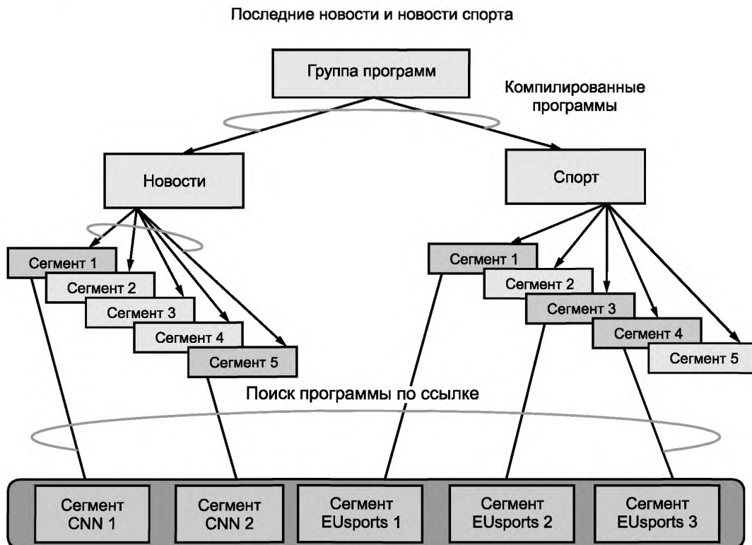
Рисунок 13 – Компиляция обновленных сегментов от нескольких провайдеров
