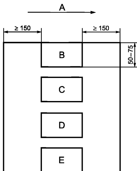
A — поперечное направление продукции; B — крайняя нарезаемая полоска; C — средняя нарезаемая полоска; D — средняя нарезаемая полоска; E — крайняя нарезаемая полоска
