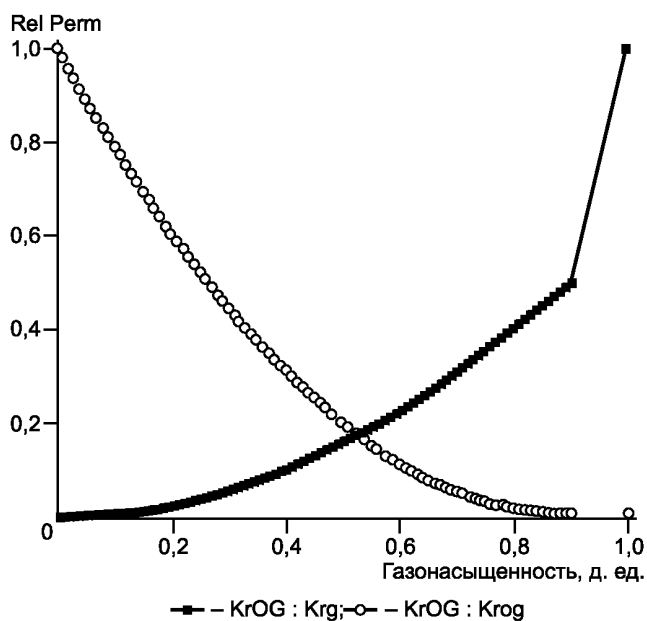
Рисунок В.3 — Относительные фазовые проницаемости
