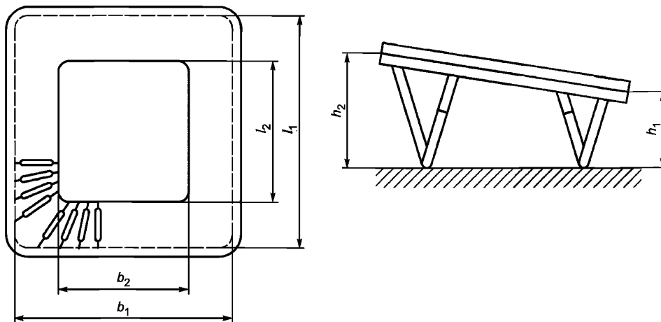
Рисунок 2 — Размеры батутов класса 2
