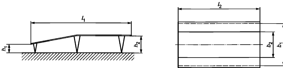
Рисунок 4 — Размеры батутов класса 4
