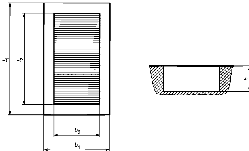
Рисунок 5 — Размеры батутов класса 5
