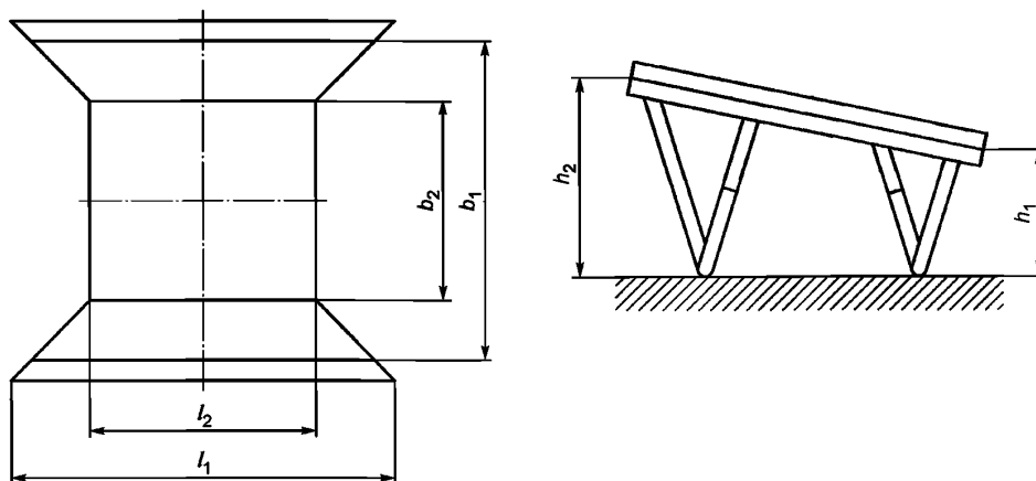
Рисунок 3 — Размеры батутов класса 3
