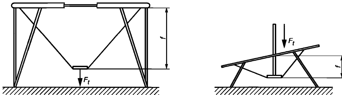
Рисунок А.1 — Схема приложения испытательной нагрузки F_t при определении упругости прыжкового полотна батута
