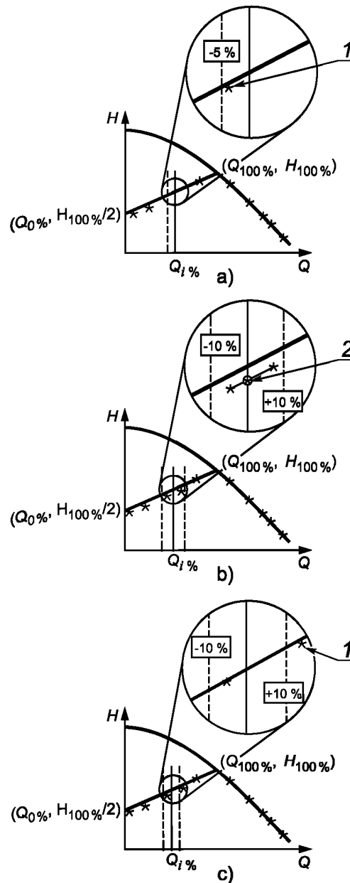
Рисунок 5 — Правила интерполяции
