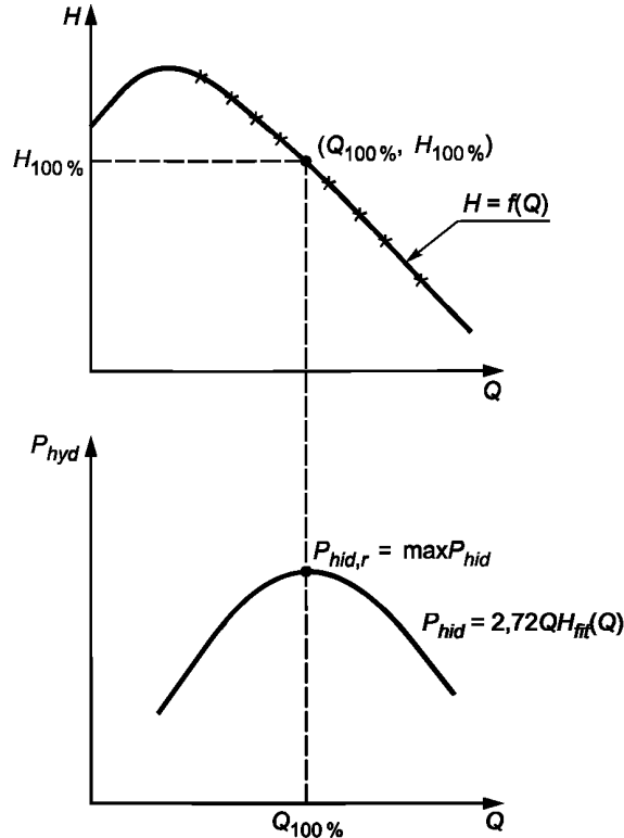
Рисунок 2 — Номинальная гидравлическая мощность на выходе
