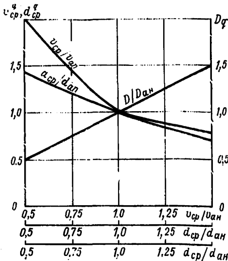
Рис. 5-1. Зависимость расчетных значений множителей для крупнокускового шлака от относительных параметров транспортирования.
