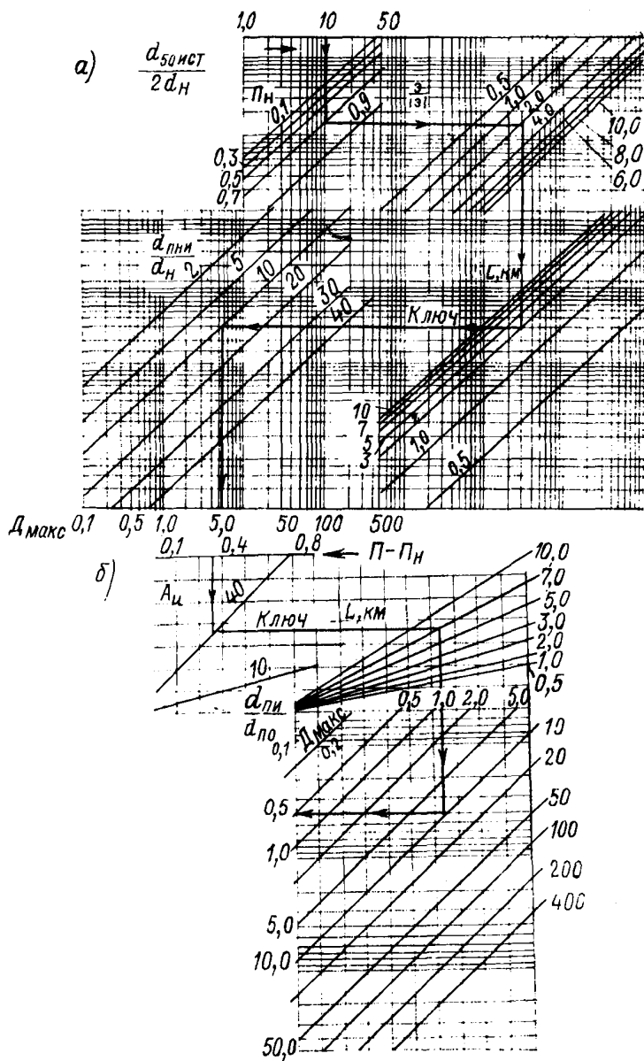
Рис. 4-3. Номограммы для определения параметра D_{\text{max}} (а) и отношения d_{\text{пл}}/d_{\text{по}} (б) для твердого шлака при известных характеристиках гранулометрического состава транспортируемого материала, параметрах потока и длине трассы пульпопровода.
