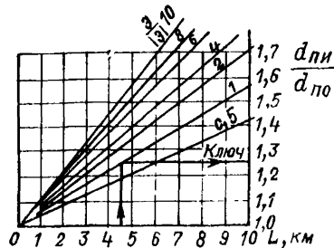
Рис. 4-2. Номограмма для определения соотношения \frac{d_{\text{пн}}}{d_{\text{по}}} при известных |Э| и длине трассы пульпопровода для жидкого шлака.
