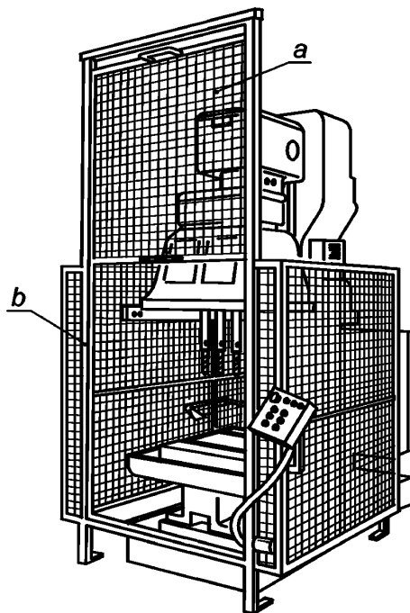
a — блокирующее защитное ограждение в открытом положении; b — блокирующее защитное ограждение с фиксацией закрытия
