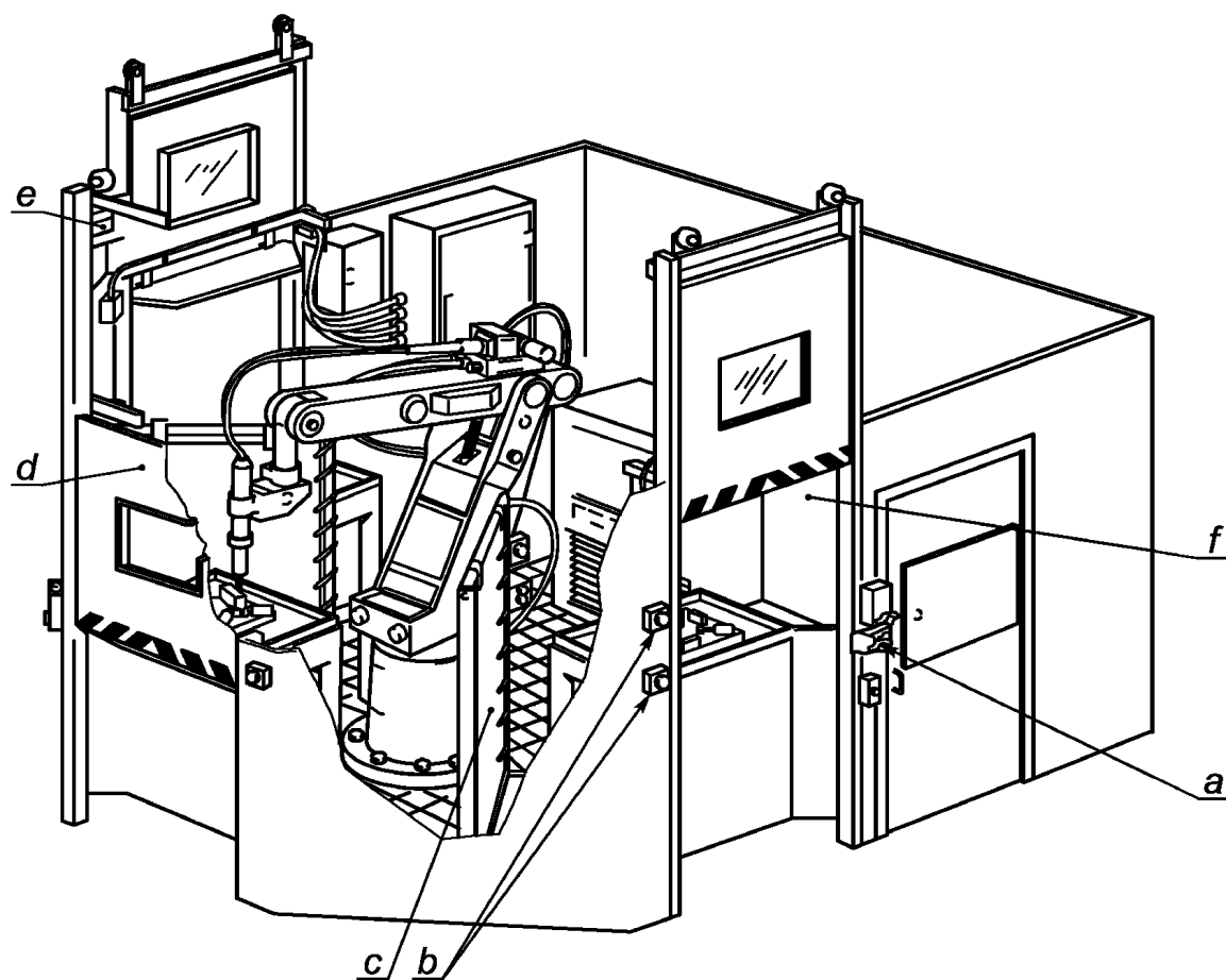
Рисунок 9 — Комбинация различных ограждений и ограждений с другими устройствами (пример 1)
