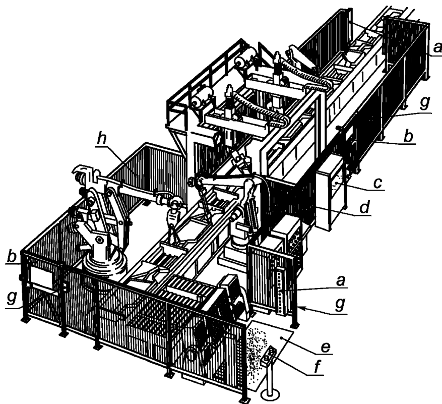
Рисунок 9 — Комбинация различных ограждений и ограждений с другими устройствами (пример 1)
