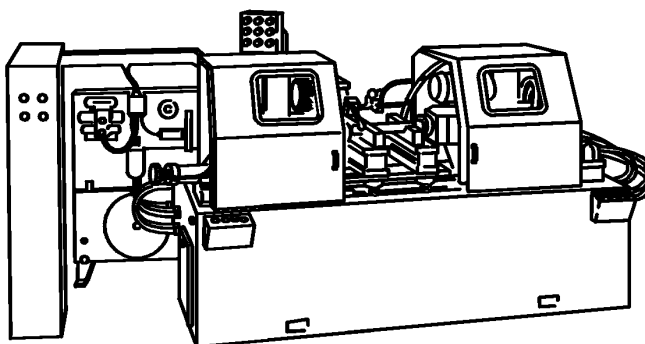
Рисунок 7 — Пример блокирующих перемещаемых защитных ограждений
