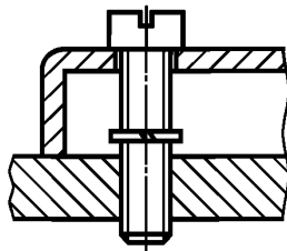
Рисунок 11 — Пример удерживаемого крепления
