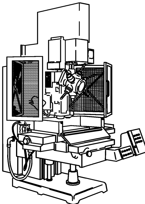
Рисунок 6 — Пример блокирующих навесных защитных ограждений, которые охватывают опасную зону при их закрытии
