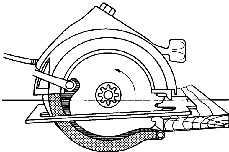
Рисунок 4 — Пример самозакрывающегося ограждения
