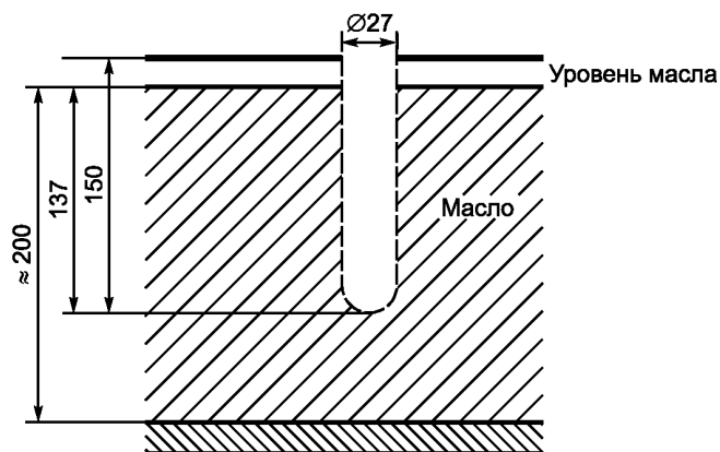
Рисунок 3 — Положение пробирки в масляной бане
