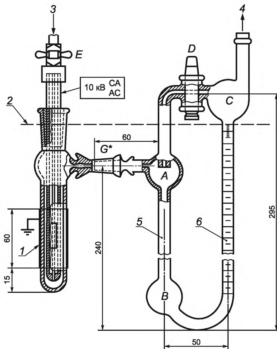
A, B, C — шарообразные расширения стеклянной трубки; D — перепускной кран; E — игольчатый вентиль; G — конусное стеклянное соединение 10/19 (по стандарту [3]); 1 — внешний электрод; 2 — уровень жидкости в масляной бане; 3 — подача газа; 4 — в атмосферу; 5, 6 — прозрачная трубка внутренним диаметром 5 мм и наружным диаметром 7 мм по стандарту [1]
