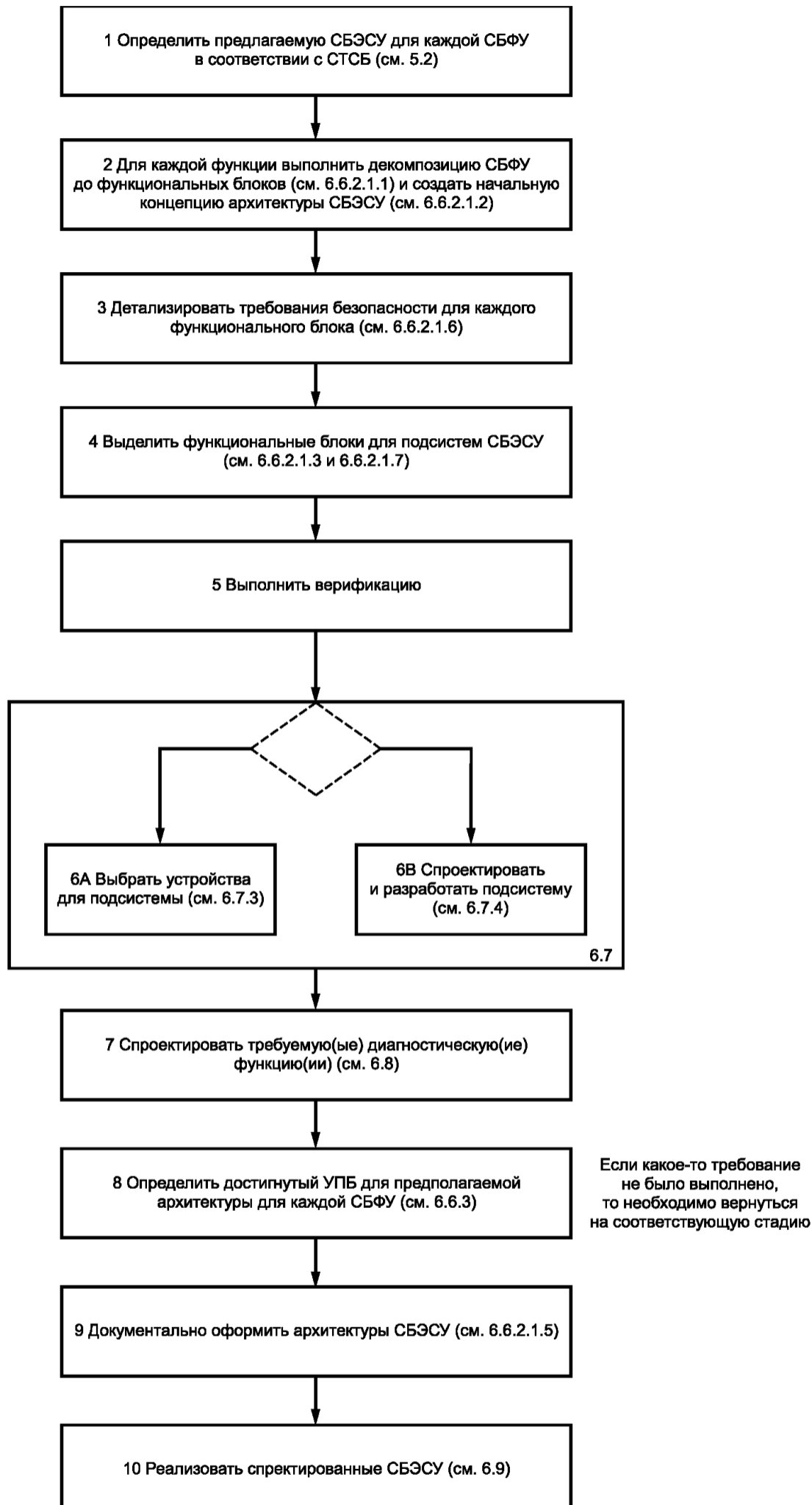
Рисунок 2 — Структура процесса проектирования и разработки СБЭСУ
