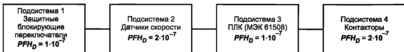
Рисунок В.8 — Оценка PFH_D для СБЭСУ
