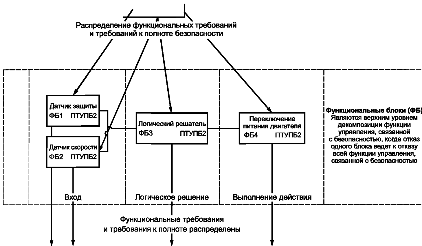
Рисунок В.5 — Начальная концепция архитектуры СБЭСУ
