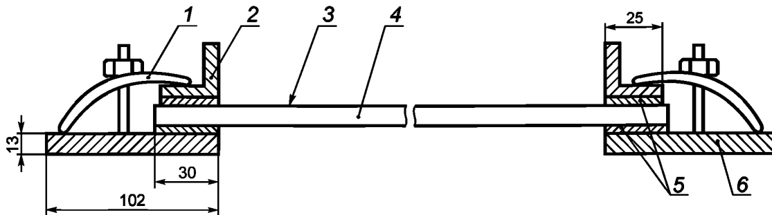
1 — зажим; 2 — внутренняя рама; 3 — поверхность остекления 900 × 1100 мм; 4 — образец; 5 — резина; 6 — наружная рама
