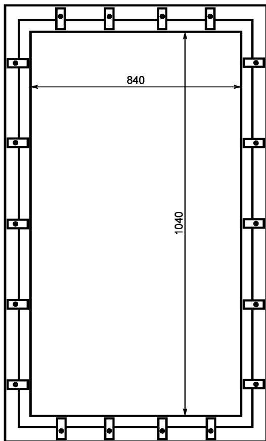
Изготовлено из стальной ленты 102 × 13 мм
