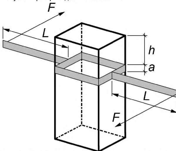
Рисунок 3— Приспособление для проведения испытания на кручение
