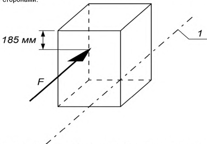
Рисунок 1 – Схема приложения нагрузки к тумбам класса ДТ1
