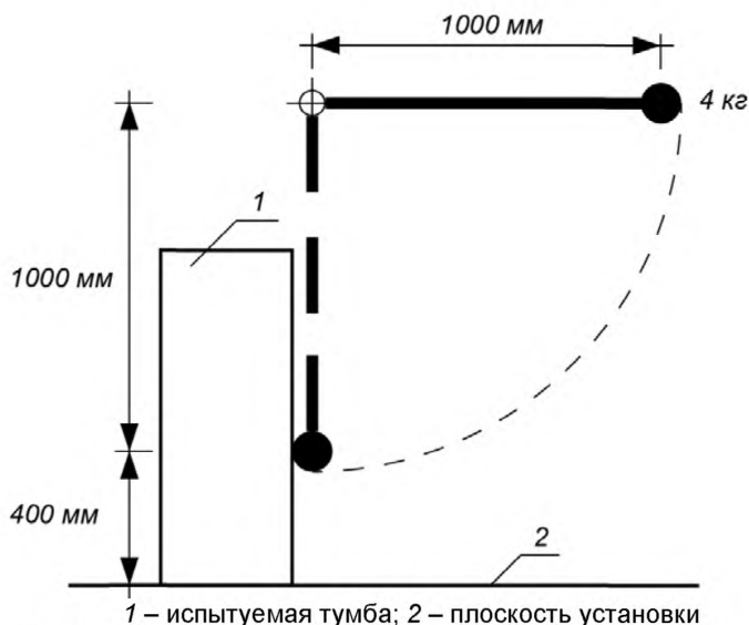
Рисунок 4 – Испытание на малую динамическую нагрузку
