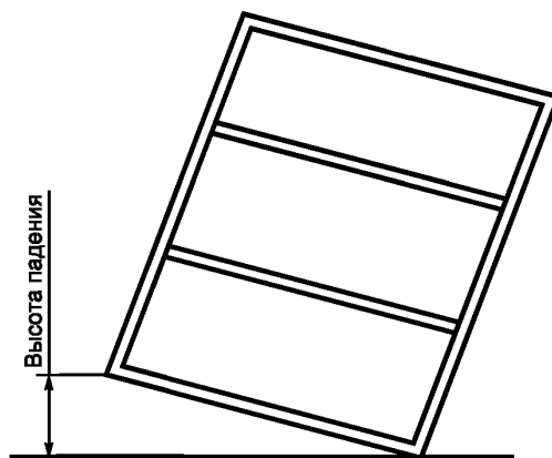
Рисунок 4 — Испытание картотек на прочность
