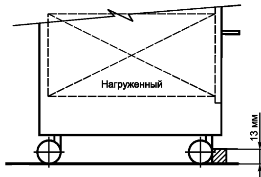
Рисунок 1 — Установка картотек для проведения испытаний
