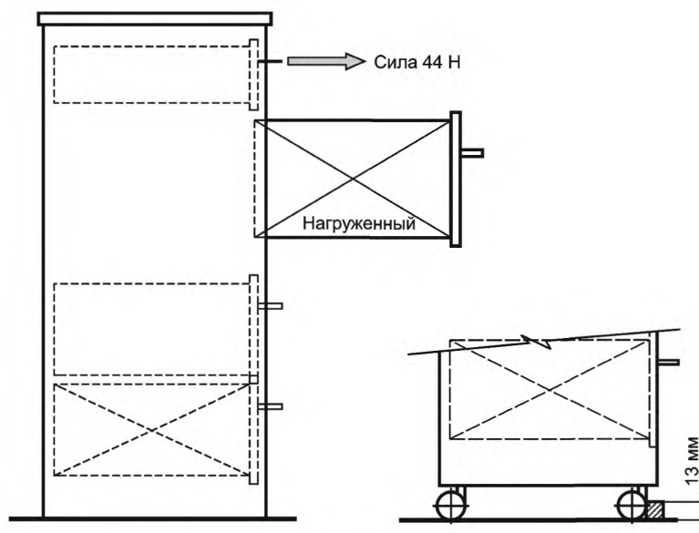
Рисунок 2 — Испытание картотек на устойчивость
