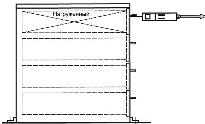
Рисунок 7 — Испытание на тянущее усилие
