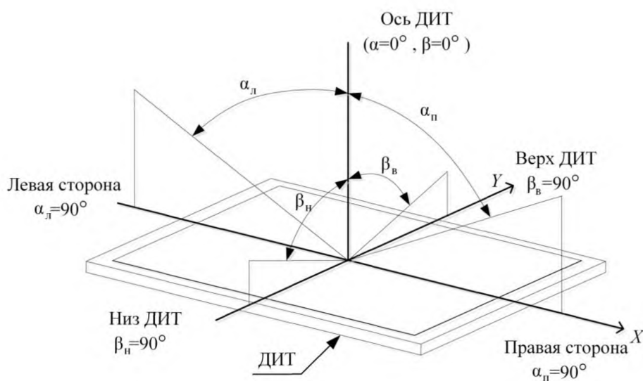
Рисунок 9.1 – Определение углов обзора
