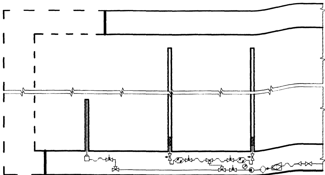
Рис. 8. Технологическая схема увлажнения очистного блока по мере его подготовки в режиме высоконапорного нагнетания жидкости насосной установкой. Бурение скважин с вентиляционного или конвейерного штрека (схема 8)
