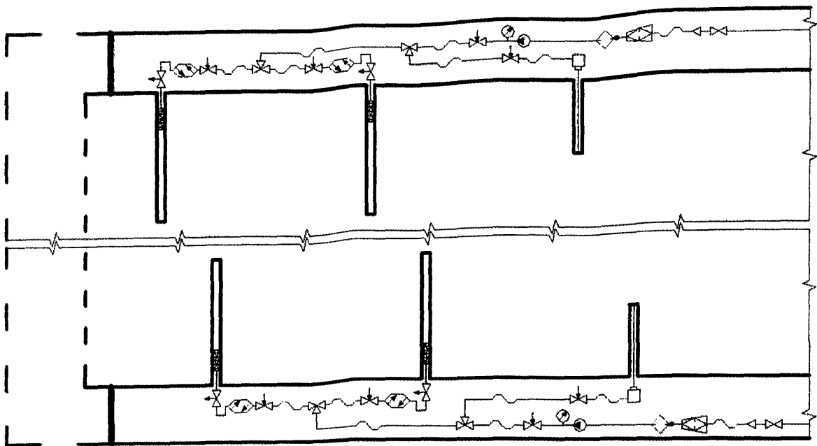
Рис. 9. Технологическая схема увлажнения очистного блока по мере его подготовки в режиме высоконапорного нагнетания жидкости насосной установкой. Бурение скважин с вентиляционного и конвейерного штрека (схема 9)
