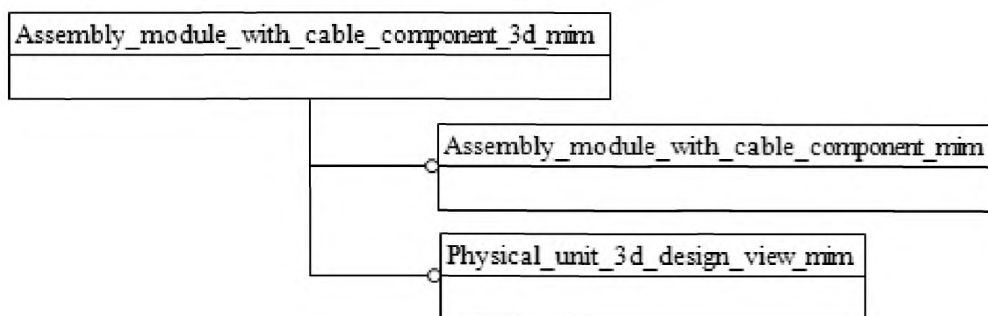
Рисунок D.1 – Представление ИММ на уровне схем в формате EXPRESS-G
