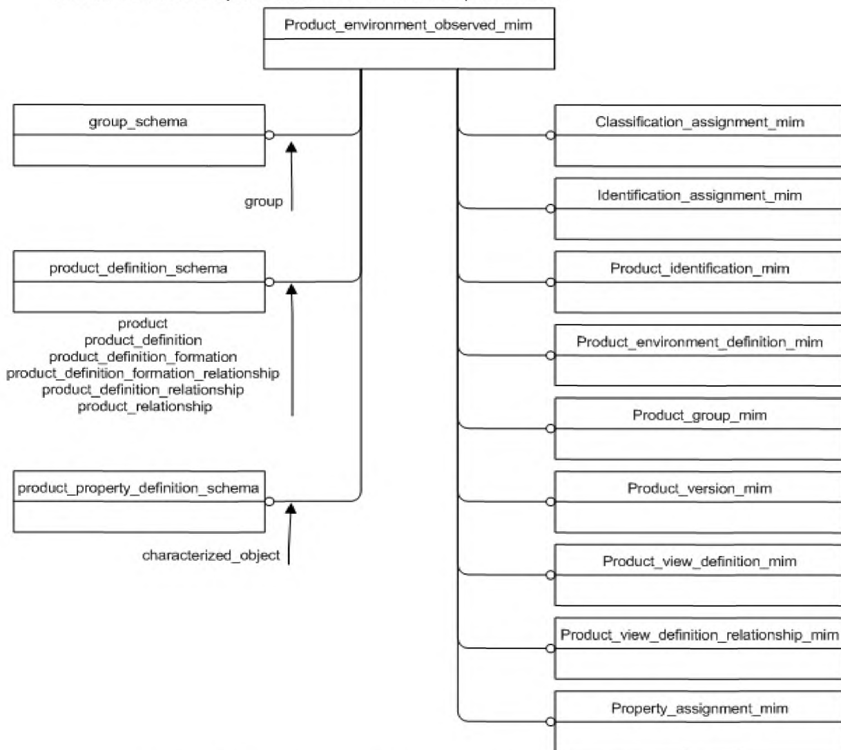
Рисунок D.1 – Представление ИММ на уровне схем в формате EXPRESS-G
