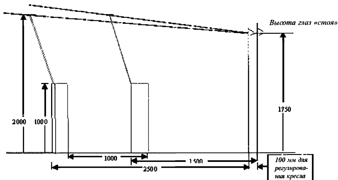
Рис. 2.6.3 При наклоне передних окон на угол 15^\circ от вертикали угол обзора 5^\circ выше горизонтали от уровня глаз стоящего человека, находящегося на высоте 1750 мм, может быть обеспечен на расстоянии 2600 мм от фронтальной стенки (лобовой переборки) с учетом наличия прохода шириной 1000 мм перед пультами рабочего поста
