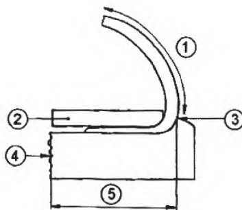
1 – ~ 15; 2 – стелька (удаленная); 3 – линия затяжной кромки; 4 – подошва; 5 – ~ 15
