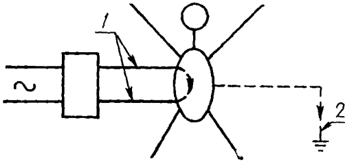
Рис. 2. Ток утечки на пациента 1 — накладываемая часть или цепь пациента; 2 — ток утечки
