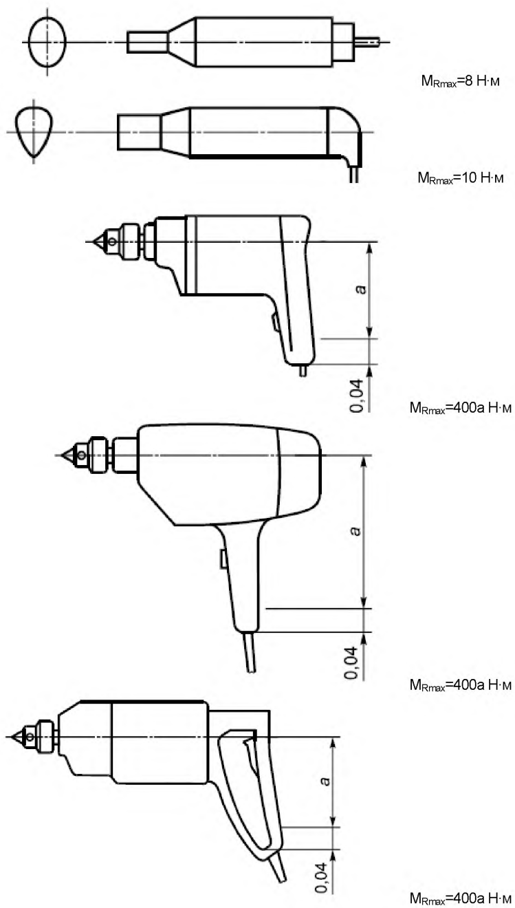
Рисунок 101 – Машины, удерживаемые одной рукой
