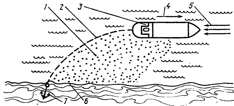
Рис. 14. Перемещение судна для увеличения ог- ражденного судном и бонами участка: 1 — нефтяное пятно; 2 — оперативные боновые загражде- ния; 3 — аварийное судно; 4 — направление передвижения судна; 5 — направление течения; 6 — линия берега; 7 — якорь
